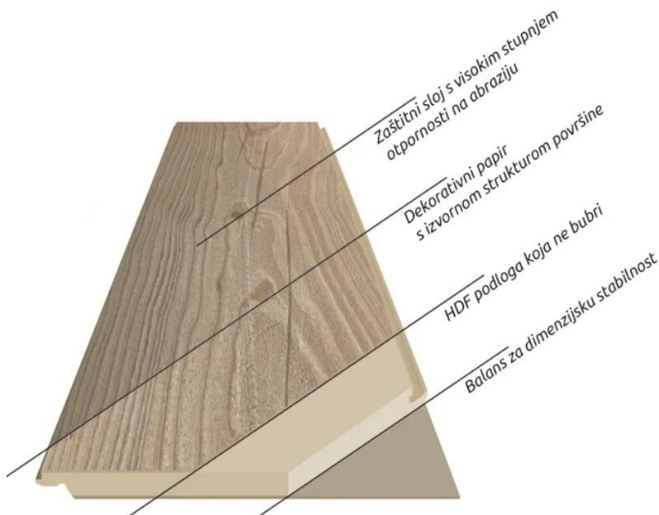
Slika 3. Slojevi laminata
