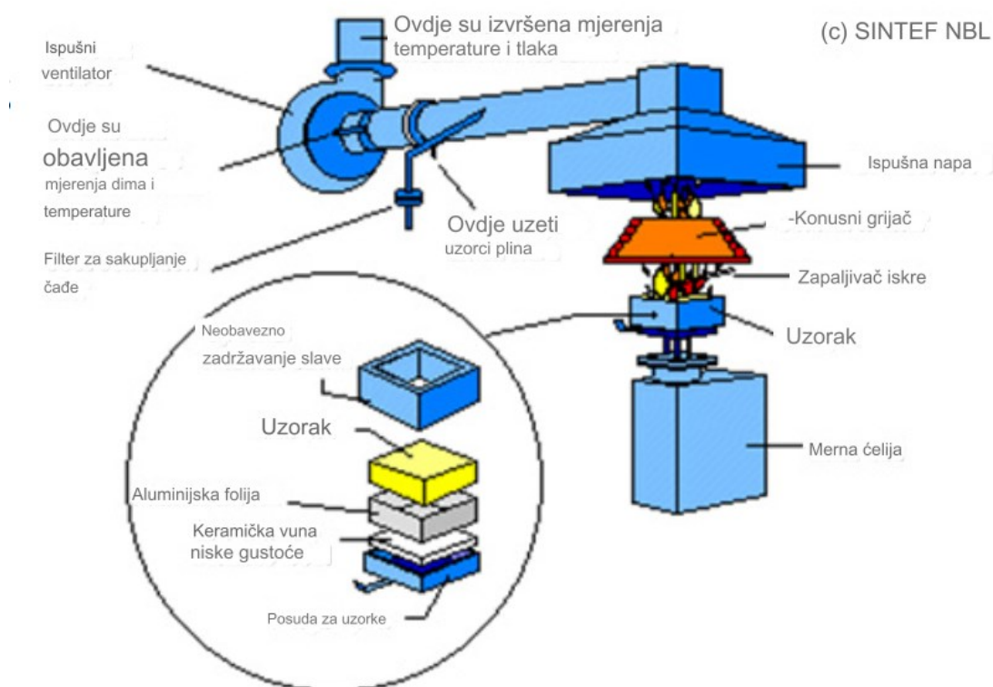
Slika 6. Konusni kalorimetar [11]
