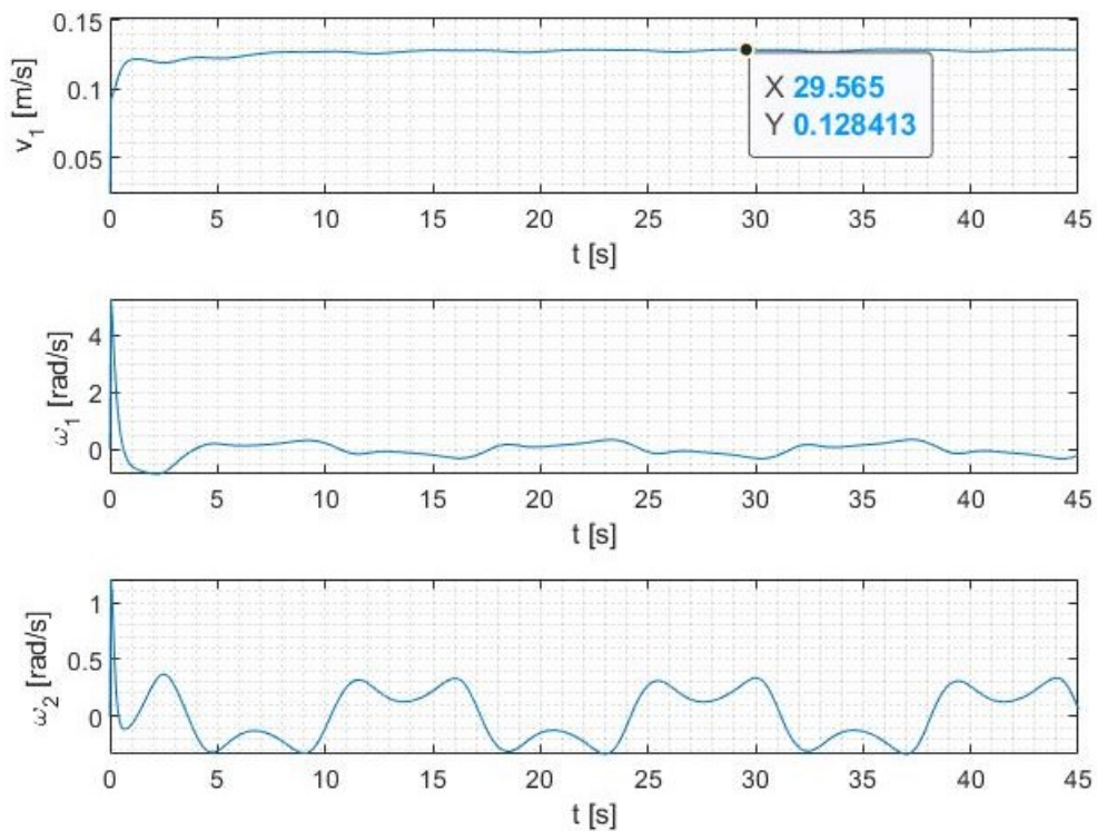
Slika 5.17: Vrijednosti upravljačkih varijabli nelinearnog modela sinusoidne trajektorije nakon ograničenja brzine
