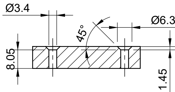
A-A (1:1)
