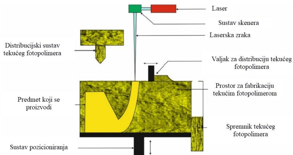
Slika 3.2 Stereolitografija [8]
