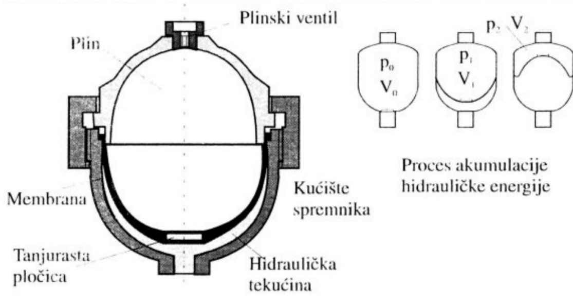
Slika 32. Hidropneumatski akumulator s membranom [11]
