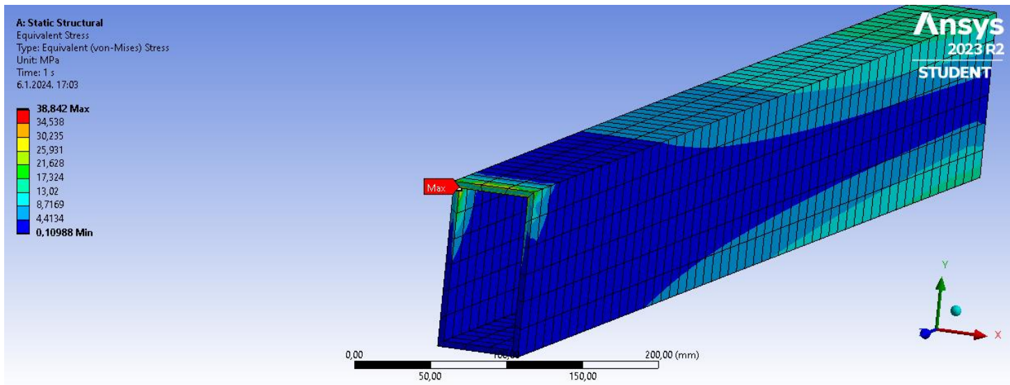
Slika 30. Prikaz ekvivalentnog naprezanja prema Von Misesu u MPa na verifikacijskom modelu u programskom paketu Ansys®
