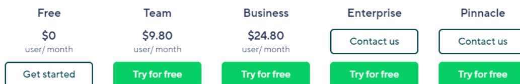
Slika 20 - Verzije Wrikea
