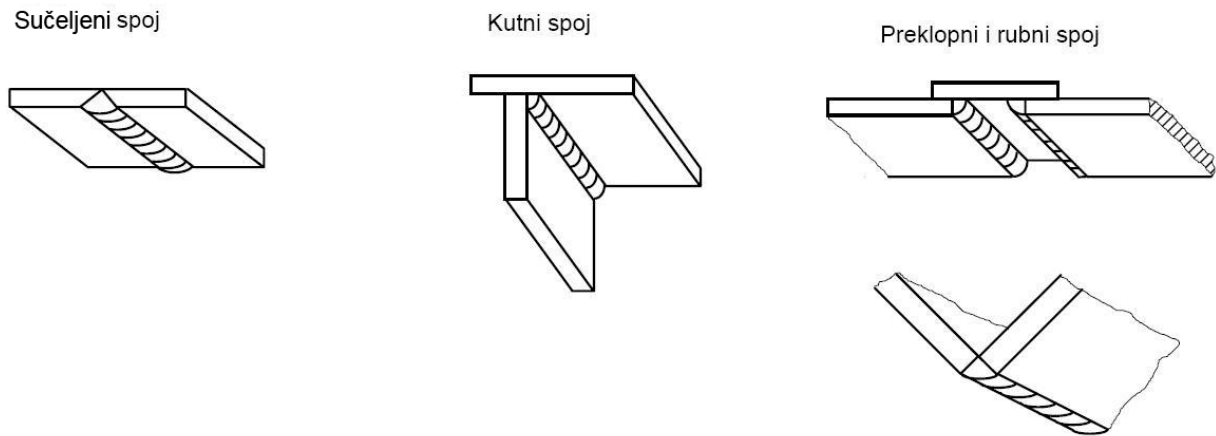
Slika 29. Nadglavni položaji zavara [16]
