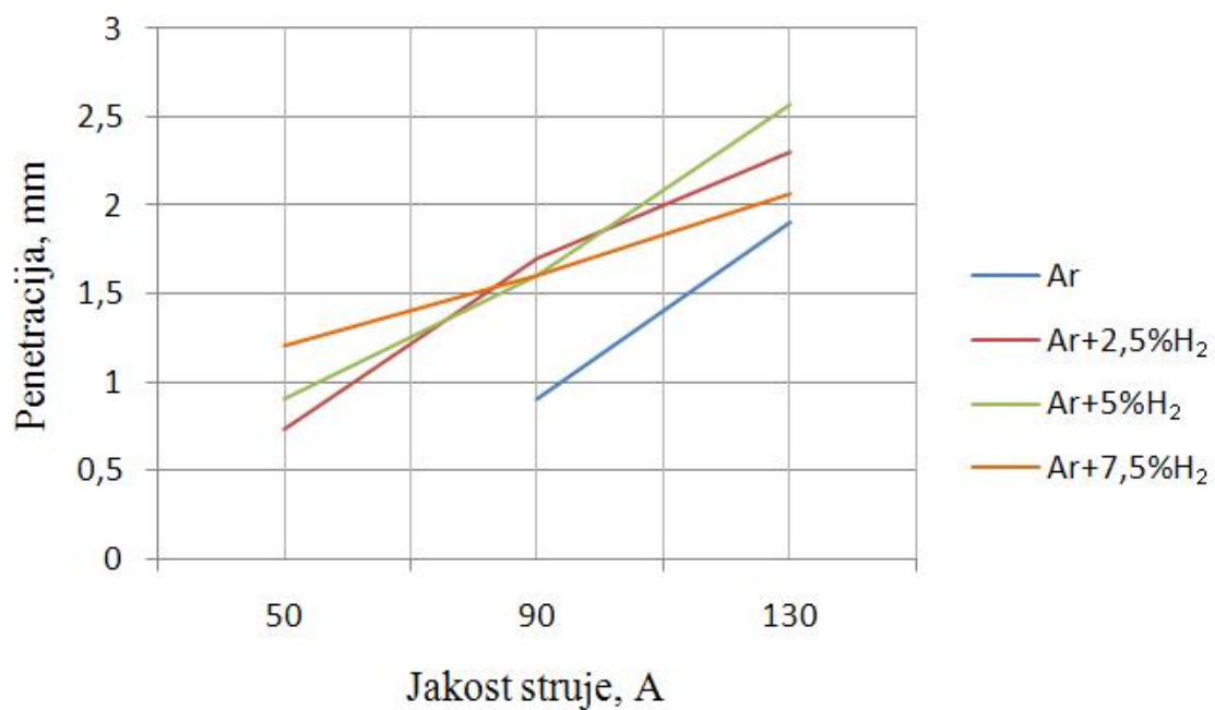
Slika 41. Utjecaj vrste zaštitnog plina na penetraciju pri navaranju impulsnim strujama
