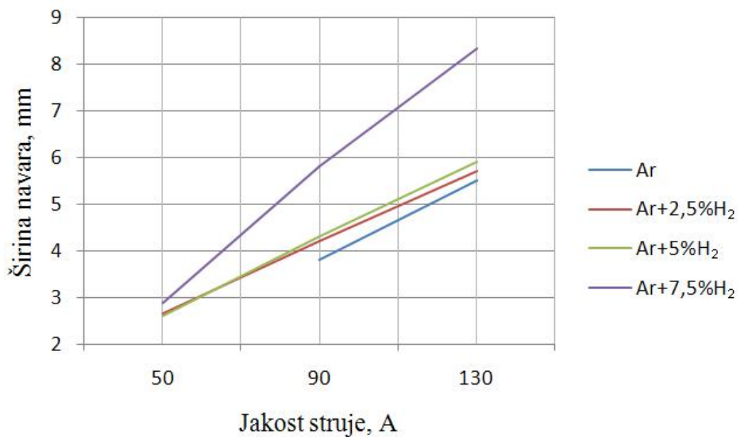
Slika 40. Utjecaj vrste zaštitnog plina na širinu navara pri navaranju kontinuiranim strujama
