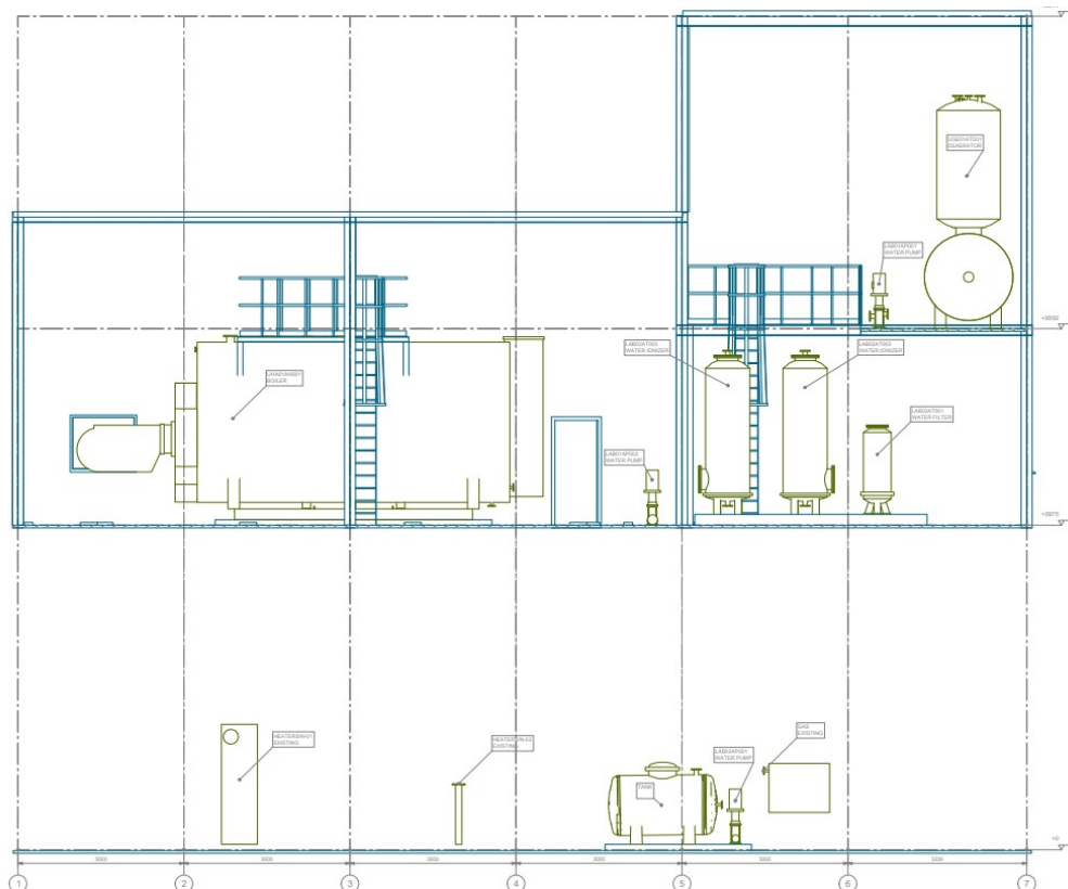
Slika 43. Plan rasporeda svih elemenata
