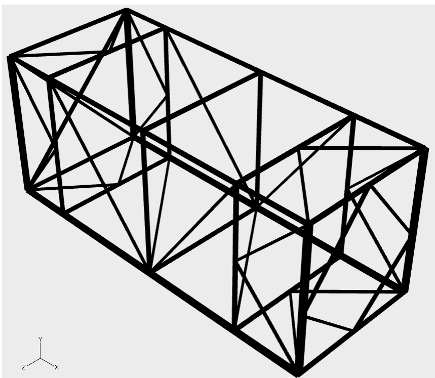
Slika 3.1 Nedeformirani oblik konstrukcijske rešetke
