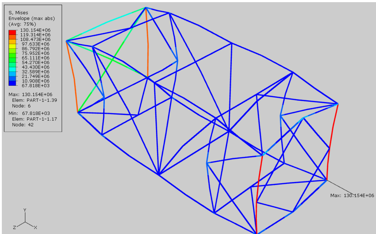
Slika 4.18 Rekonstruirana rešetka - prikaz maksimalnih ekvivalentnih naprezanja – djelovanje sila kod slaganja kontejnera jedan ma drugi
