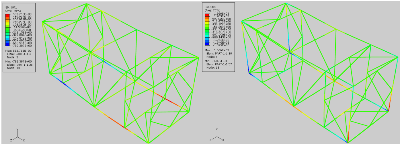
Slika 3.14 Raspodjela momenata savijanja izraženih u njutn metrima [Nm]
