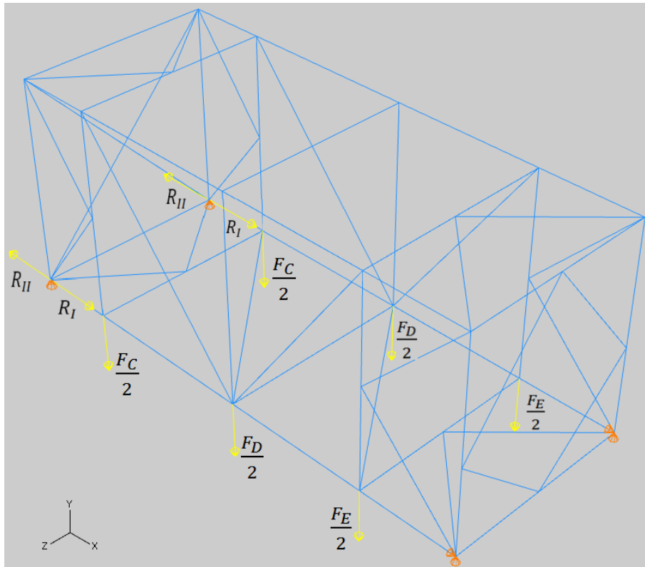
Slika 1.8 Oslanjanje na donje nauglice uz djelovanje horizontalne sile R na donjim nauglicama
