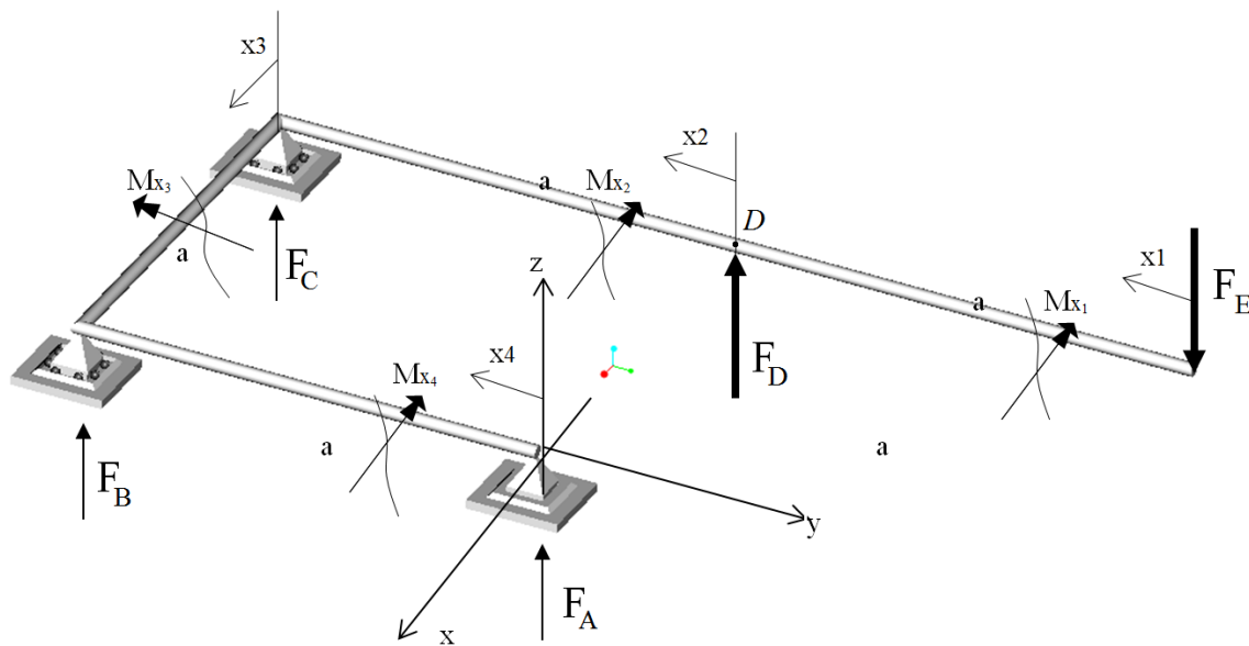
Slika 2.3 Skica trećeg primjera
