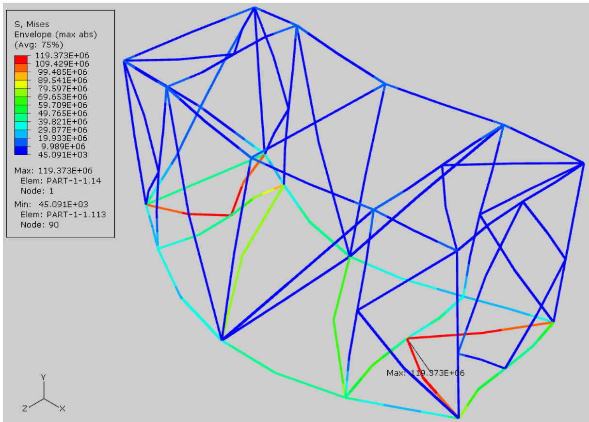
Slika 4.17 Rekonstruirana rešetka - prikaz maksimalnih ekvivalentnih naprezanja – djelovanje bočne inercijske sile na podnu rešetku I
