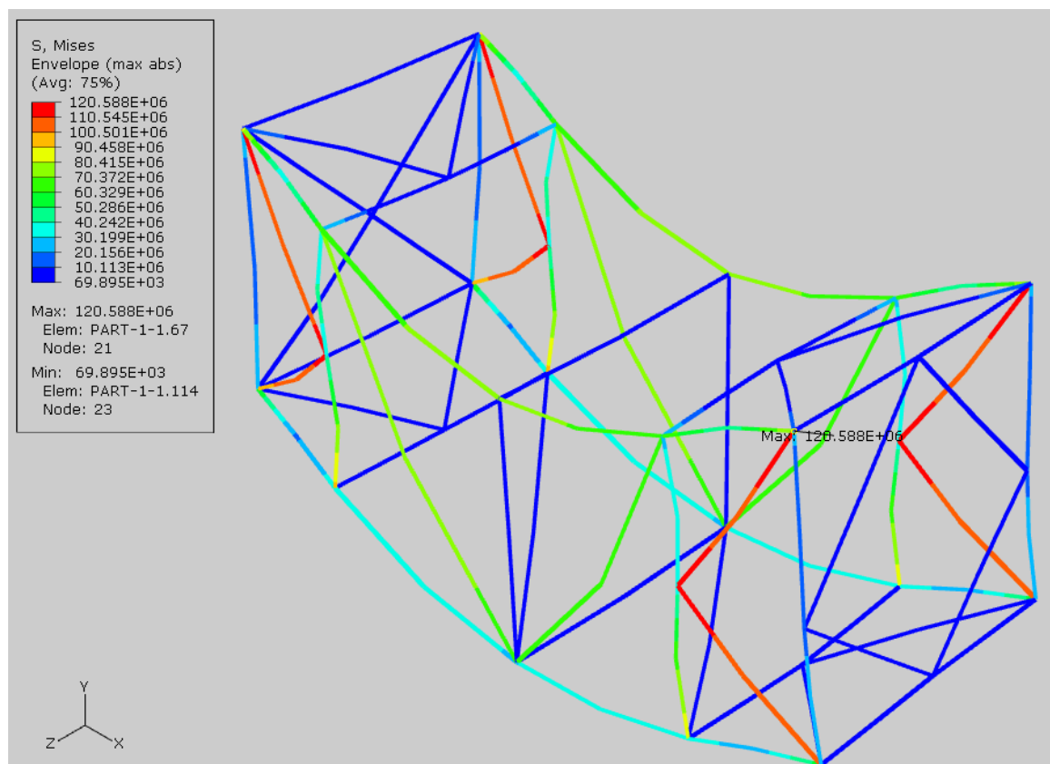
Slika 4.2 Rekonstruirana rešetka - prikaz maksimalnih ekvivalentnih napreznanja - podizanje za gornje nauglice
