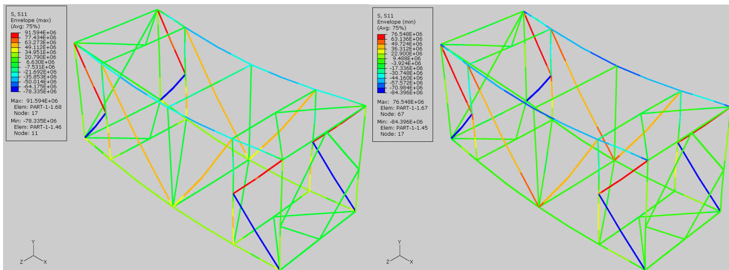
Slika 3.5 Raspodjela maksimalnih (lijevo) i minimalnih (desno) osnih napreznja po presjeku izražena u paskalima [Pa]
