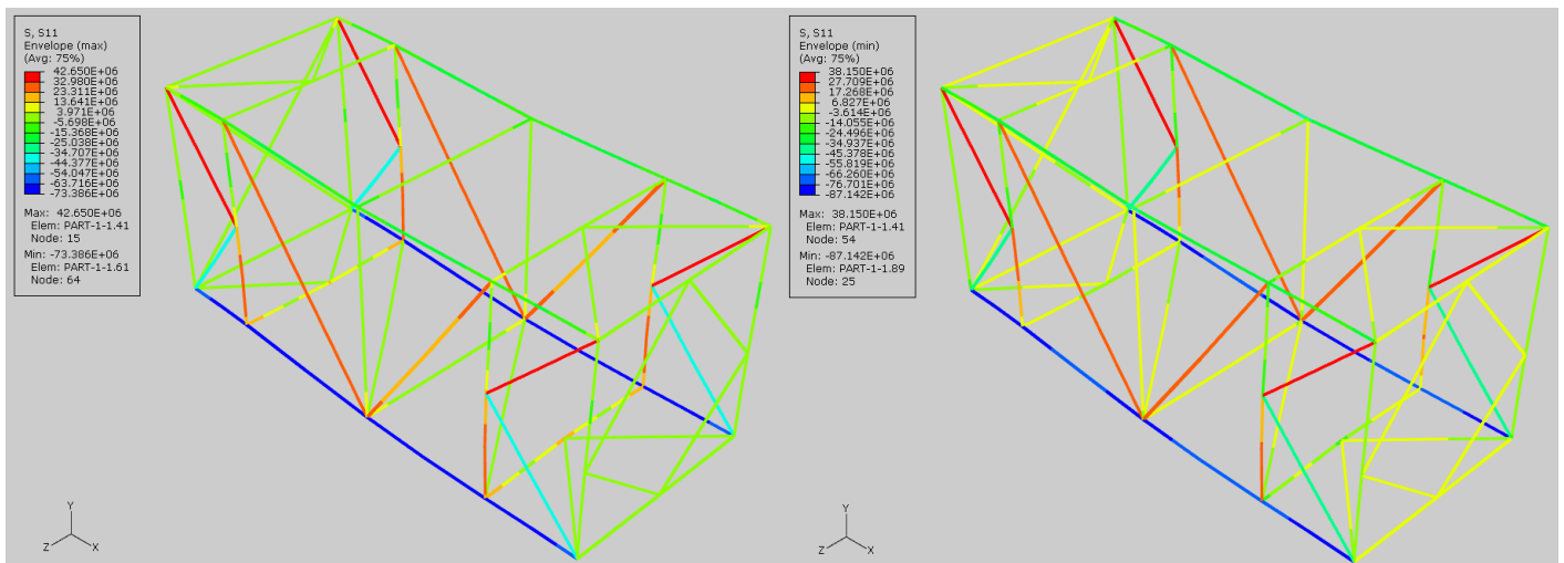
Slika 3.13 Raspodjela maksimalnih (lijevo) i minimalnih (desno) osnovih naprezanja po presjeku izražena u paskalima [Pa]
