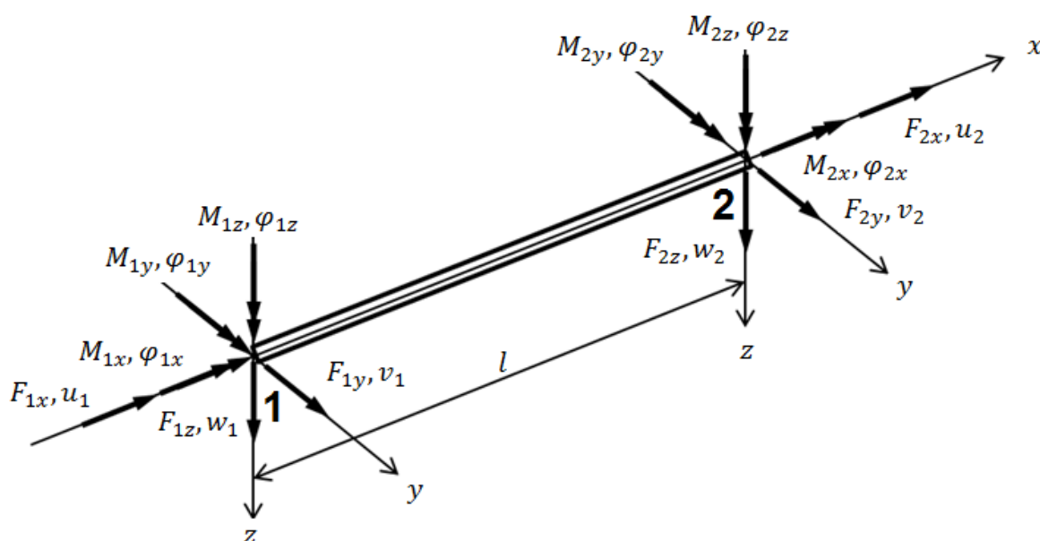
Slika 1.10 Prostorni konačni gredni element
