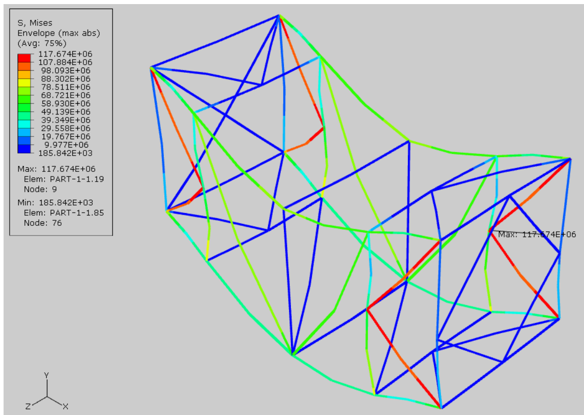
Slika 4.1 Rekonstruirana rešetka - prikaz maksimalnih ekvivalentnih napreznanja - podizanje za donje nauglice
