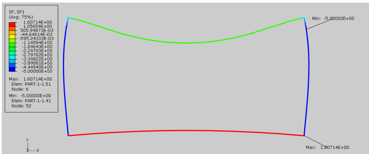
Slika 2.7 Raspodjela osne sile na deformiranom obliku
