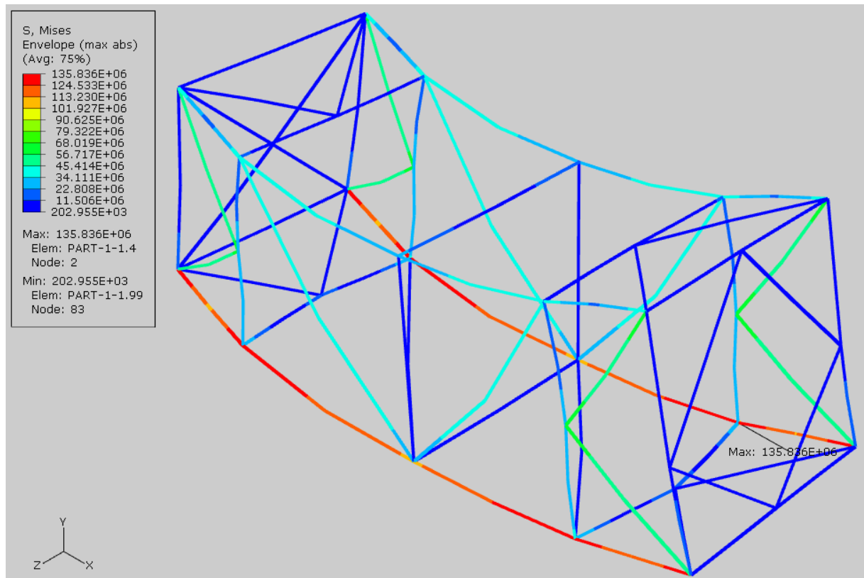
Slika 4.5 Rekonstruirana rešetka - prikaz maksimalnih ekvivalentnih napreznaja – djelovanje horizontalne vlačne sile R
