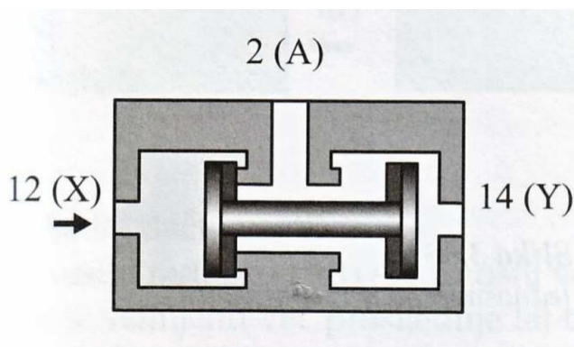
Slika 41. Skica I ventila [26]
