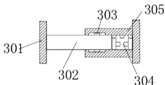
Slika 28. Prigušna šipka [21]
