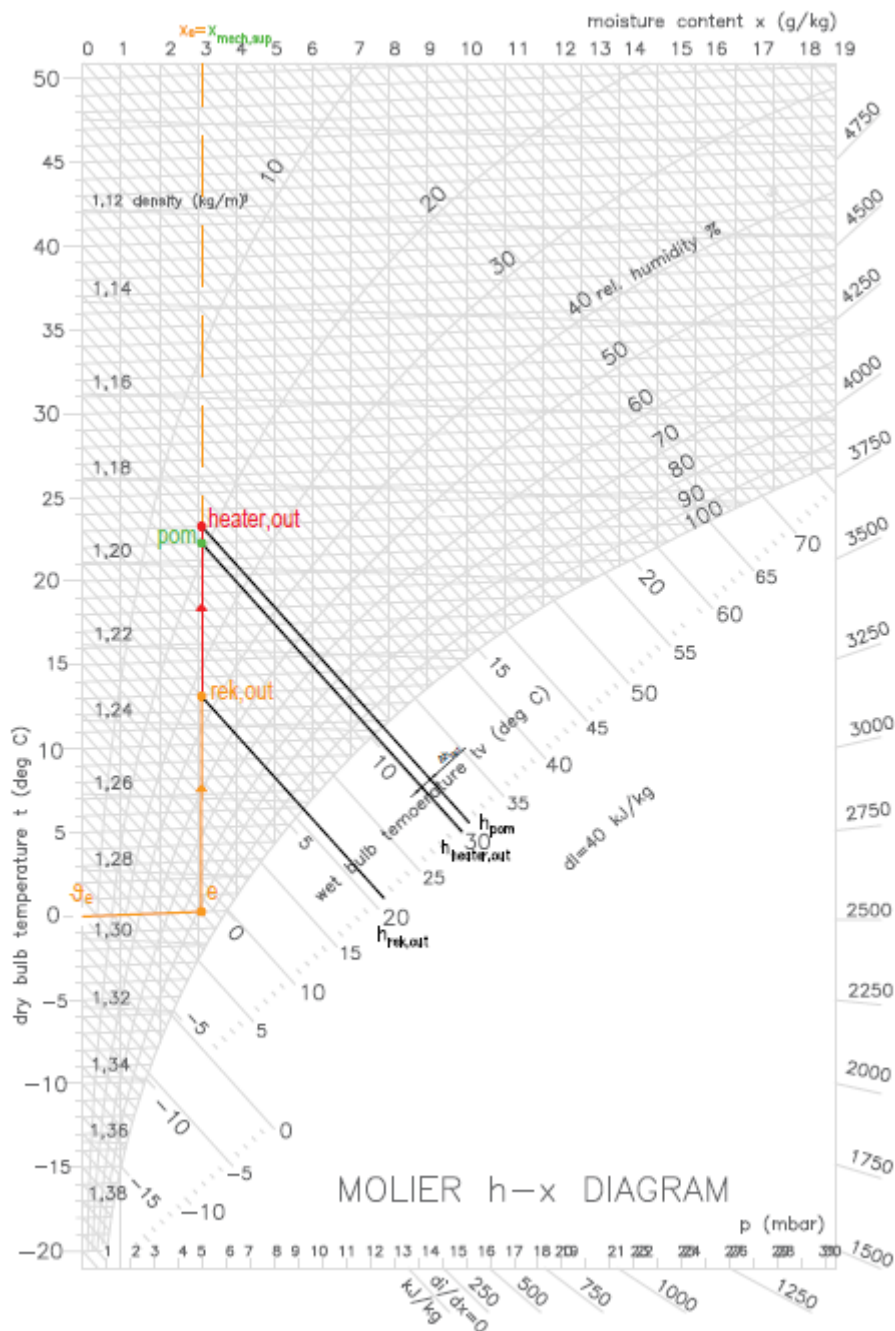
Slika 15. Proces kondicioniranja zraka u zimskom periodu za shemu 8
