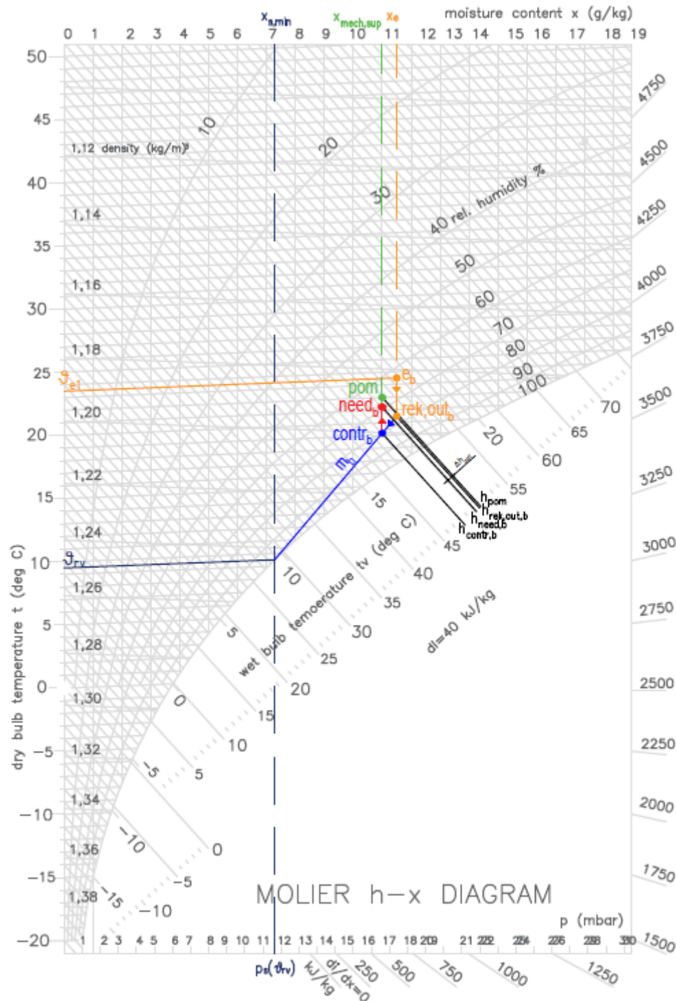
Slika 21. Proces kondicioniranja zraka ljetnom razdoblju za shemu 10 za uvjete x_e > x_{mech,sup} i h_{contr} < h_{need}
