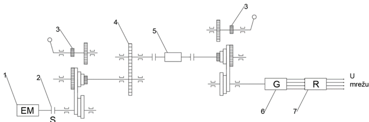
Slika 37. Koncept 2
