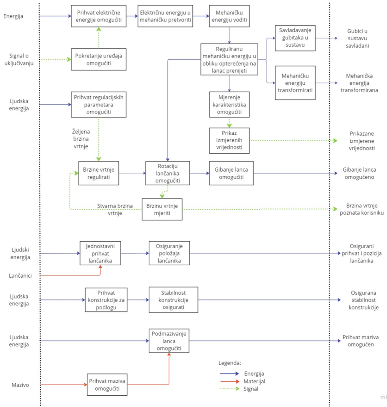
Slika 35. Funkcijska dekompozicija
