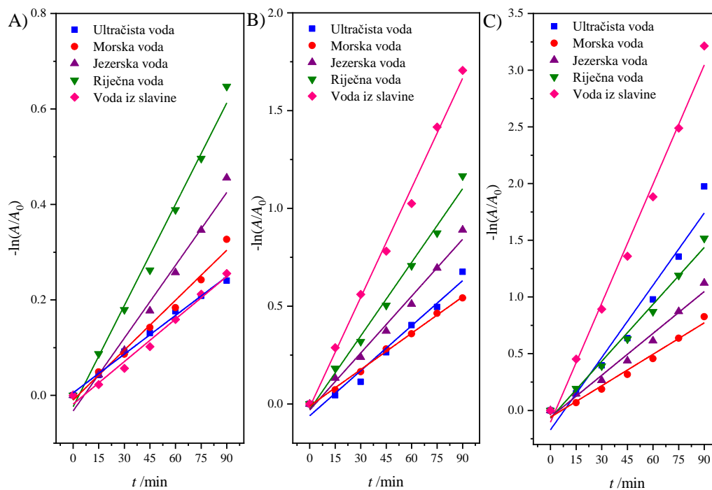
Prilog 11. Promjena relativne apsorbancije metilenskog modrila u ovisnosti o vremenu razgradnje primjenom A) fotolize, B) TiO 2 i C) TiO 2 @rGO_8 mas.%.
