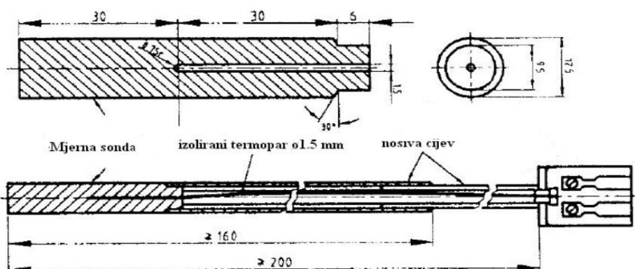
Slika 14. Shematski prikaz mjerne probe za ispitivanje krivulja
