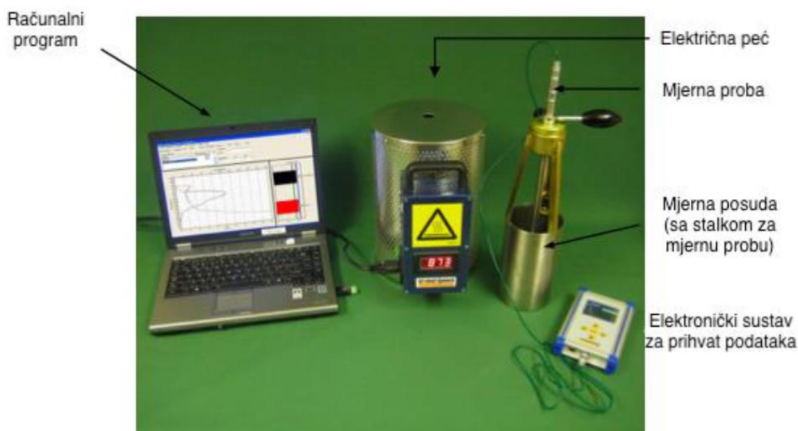
Slika 13. Mjerni sustav IVF Smart Quench za ispitivanje[17]
