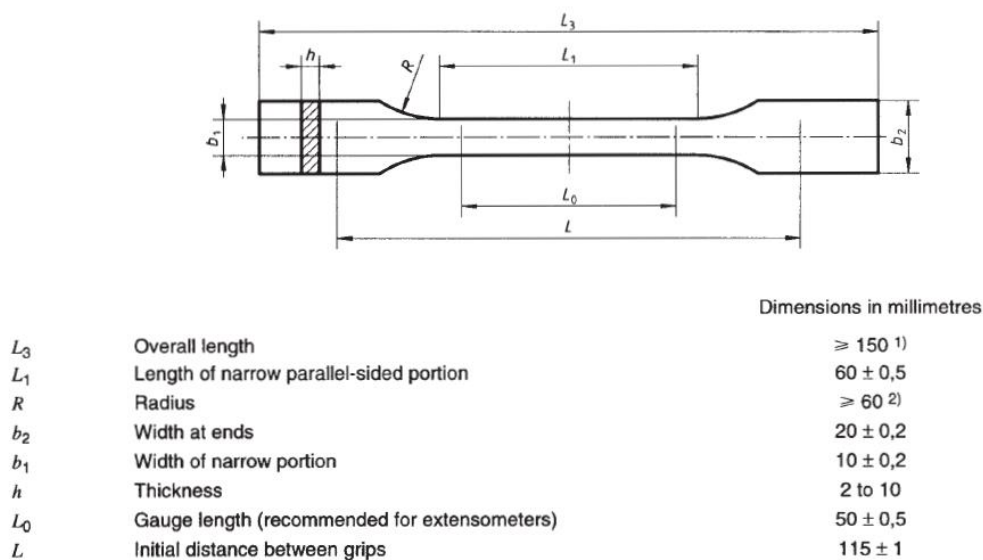
Slika 5.3 Dimenzije epruvete za vlačni test [27]
