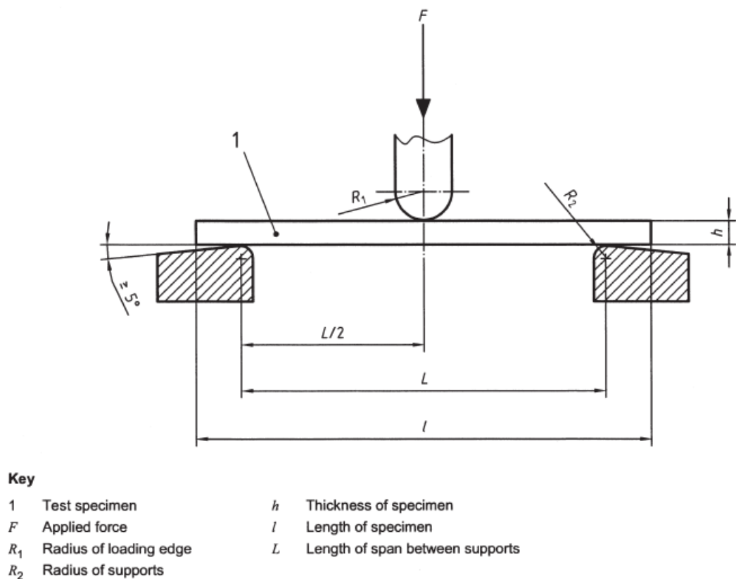
Slika 5.7 Ispitni postav za savojno ispitivanje [28]
