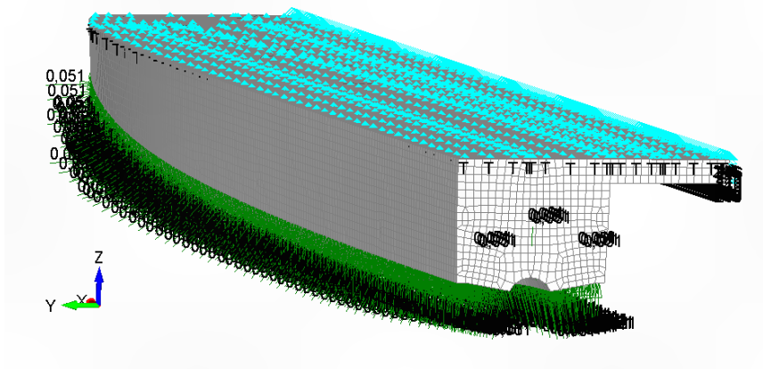
Slika 7.25 Rubni uvjeti provjere hidrostatskog tlaka na panele dna
