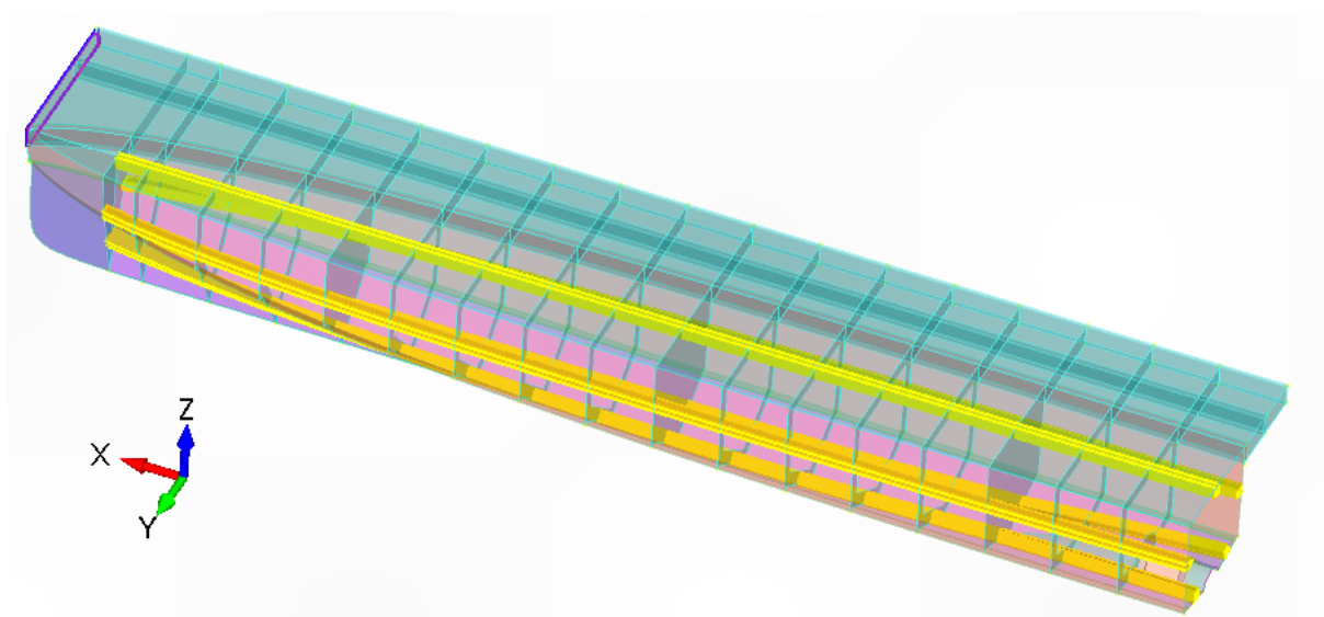
Slika 7.10 Ucrtane plohe oplata palube
