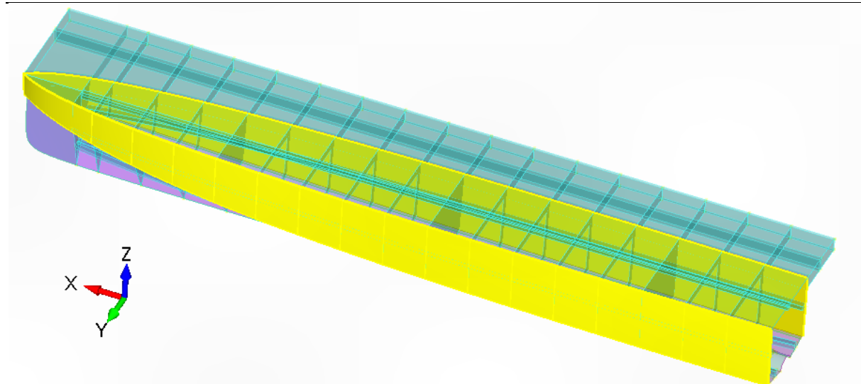
Slika 7.7 Oplata boka
