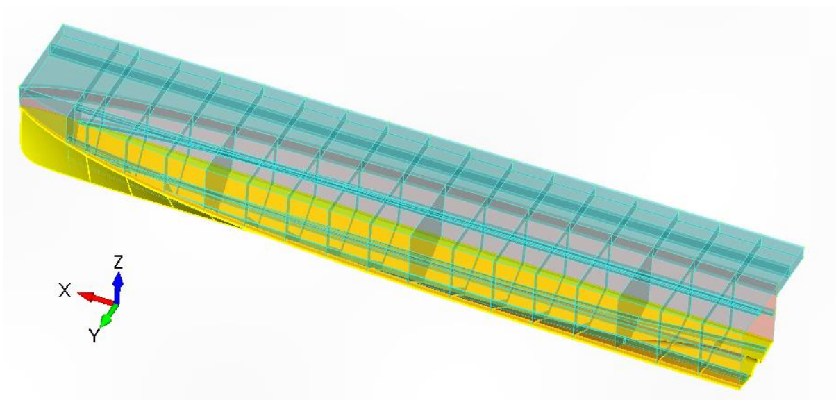
Slika 7.6 Oplata dna
