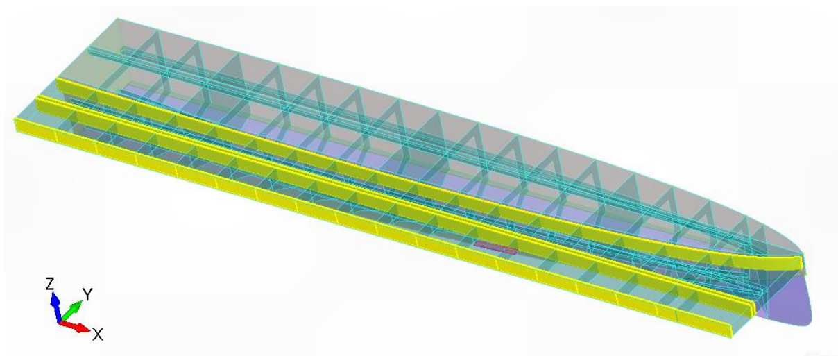
Slika 7.12 Ucrtani uzdužnjaci palube 300x100mm
