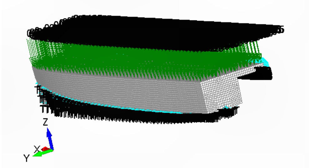
Slika 7.31 Rubni uvjeti kod hidrostatskog opterećenja palube
