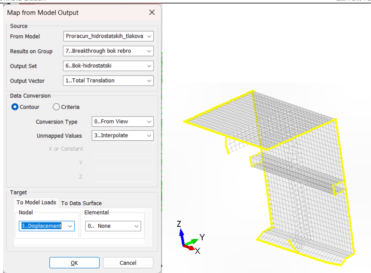
Slika 8.5 Lijevo: Izbornik prenošenja pomaka sa globalnog na izdvojeni model
