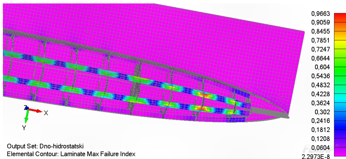
Slika 7.26 Najveći indeks popuštanja u uzdužnjacima dna pri hidrostatskom tlaku
