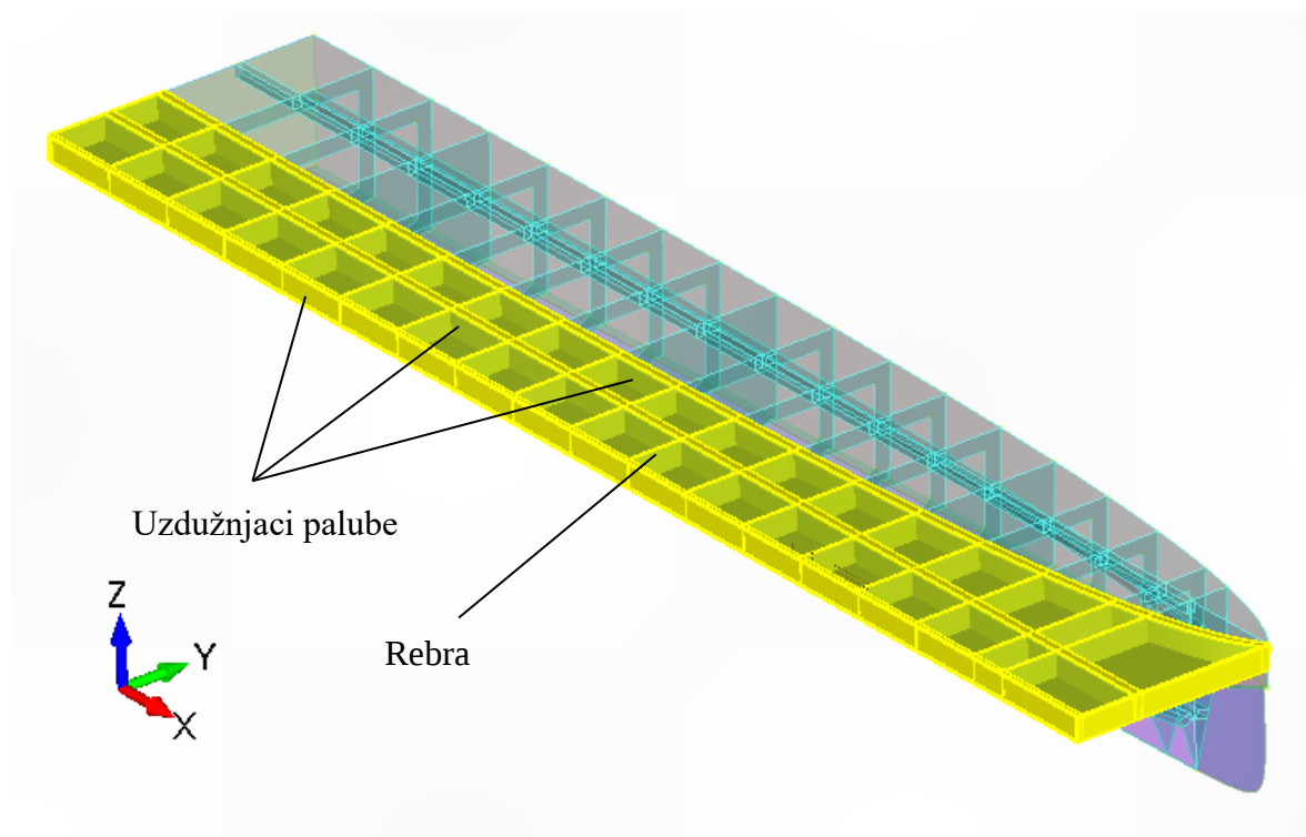
Slika 2.3 Prikaz strukture palube bez gornje oplate
