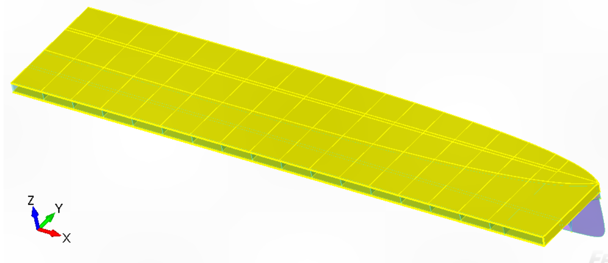
Slika 7.10 Ucrtane plohe oplata palube
