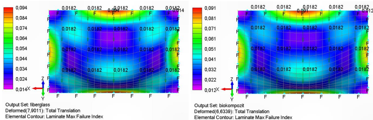
Slika 6.6 Najveći indeksi popuštanja na panelu nepropusne pregrade
