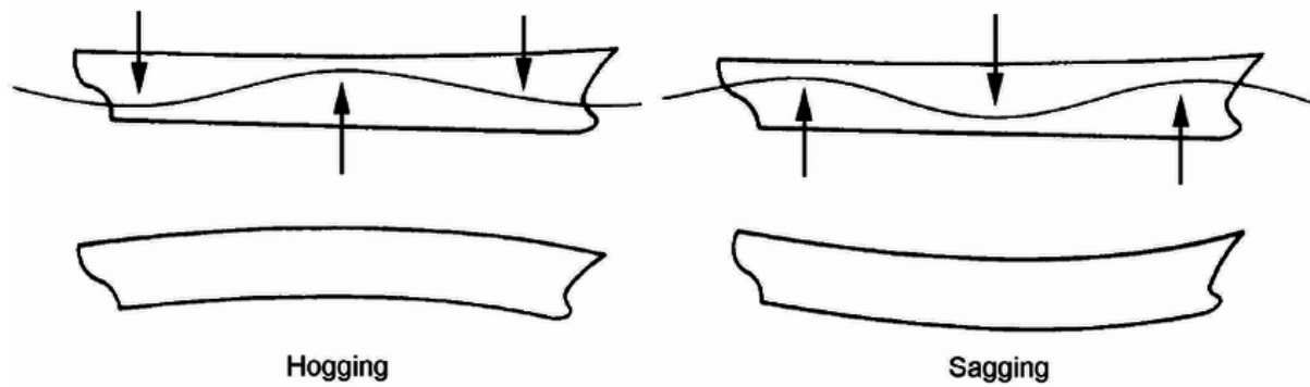
Slika 7.15 Skica progiba i pregiba broda [30]
