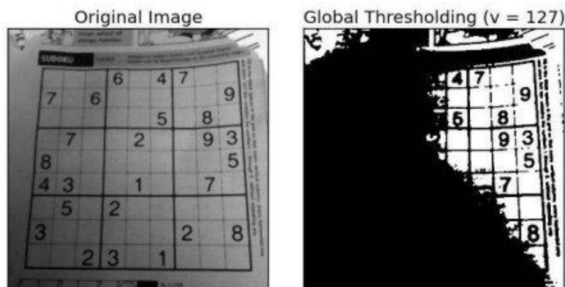
Slika 12. Rezultat thresholdanja
