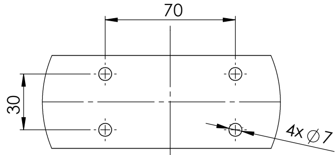
Detalj A 1 : 2
