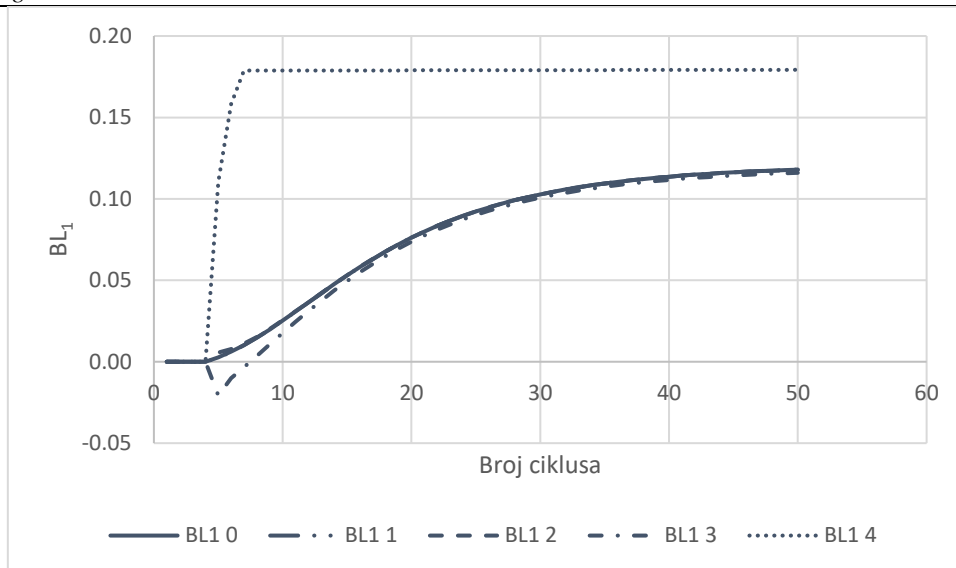
Dijagram 5.60, BL stroja 1 računat metodom konačnih stanja za slučaj D
