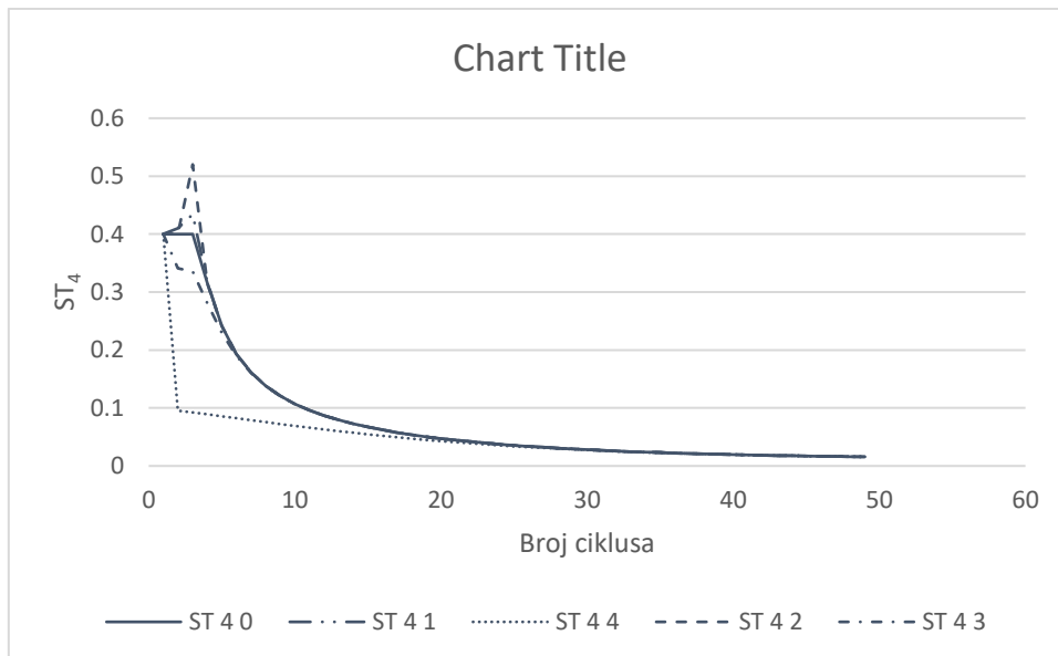
Dijagram 5.65, ST stroja 4 računat analitičkom metodom za slučaj D
