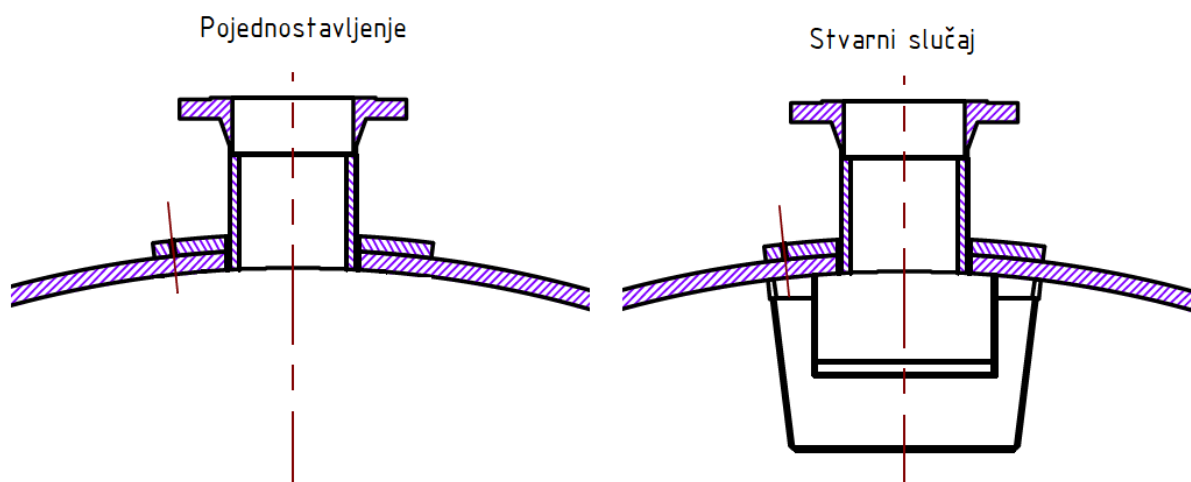
Slika 33 - Pojednostavljene prikločke za izlaz suhozasićene pare
