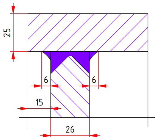
Slika 26 - Detalj zavora cilindričnog plašta i prednje cijevne stijene
