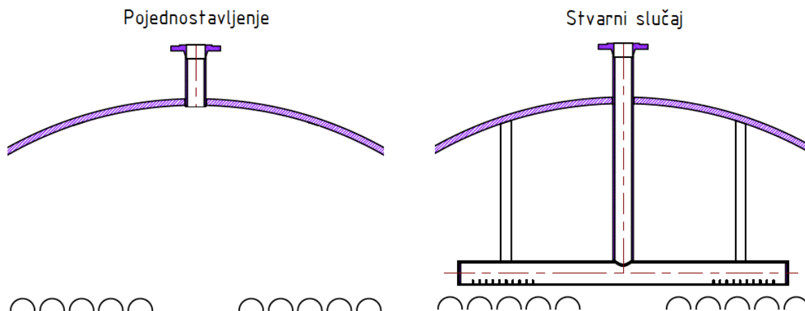
Slika 32 – Pojednostavljene prikločke za ulaz napojne vode
