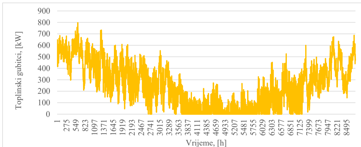
Slika 25. Ventilacijski gubitci
