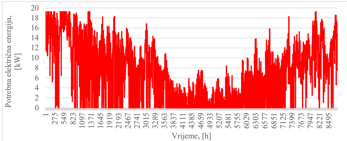
Slika 29. Potrošnja električne energije sustava za grijanje
