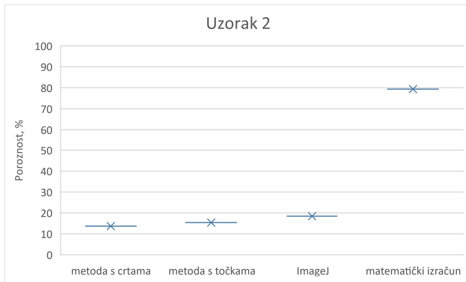
Slika 144 Poroznost uzorka 2
