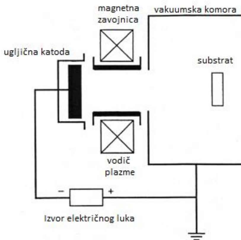
Slika 37: Jednostavni filter makro čestica sa katodom smještenom iza magnetna [3]
