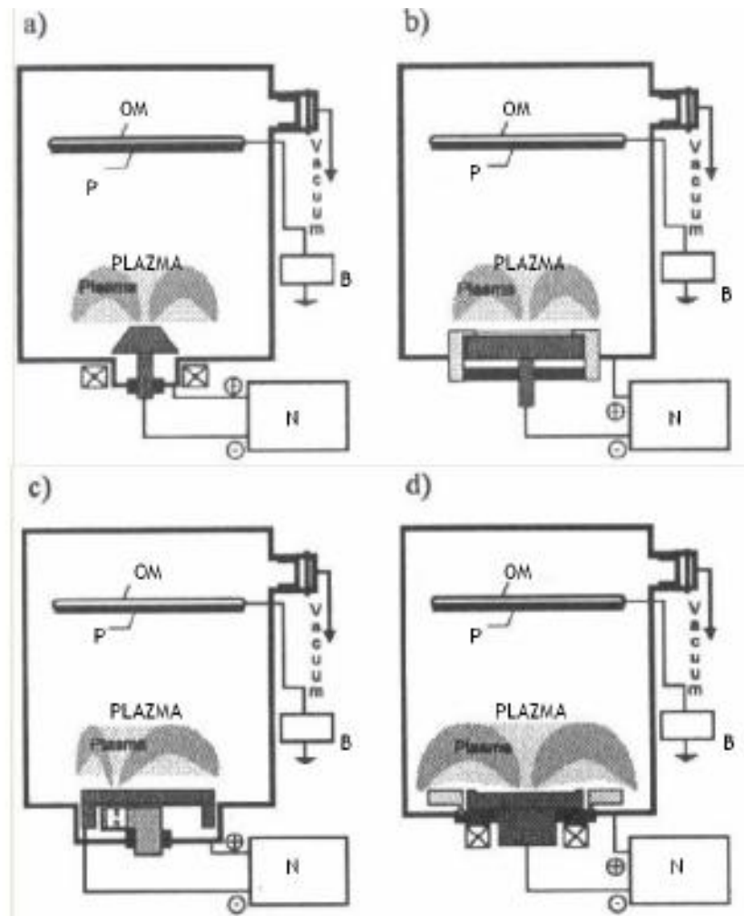
Slika 16: Shematski prikaz četiri osnovne izvedbe suustava za PVD postupak isparavanja materijala prevlake katodnim lukom: a) elektrostatski, b) elektromagnetski, c) elektromagnetski s pomičnim magnetima, d) elektrostatski-elektromagnetski [2]
