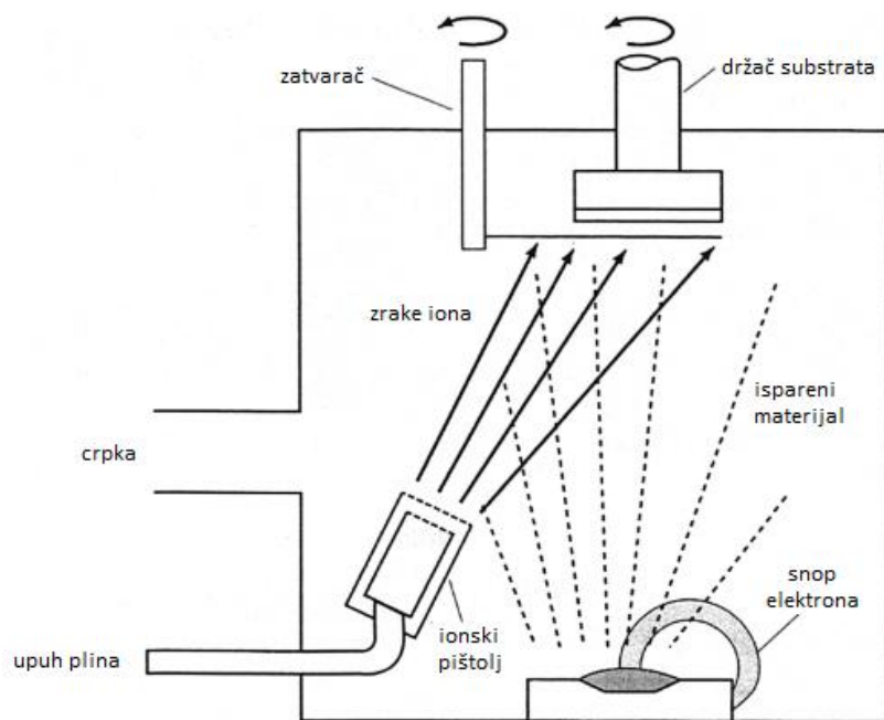
Slika 32: Shematski prikaz sustava za vakuurno ionsko platiniranje [3]
