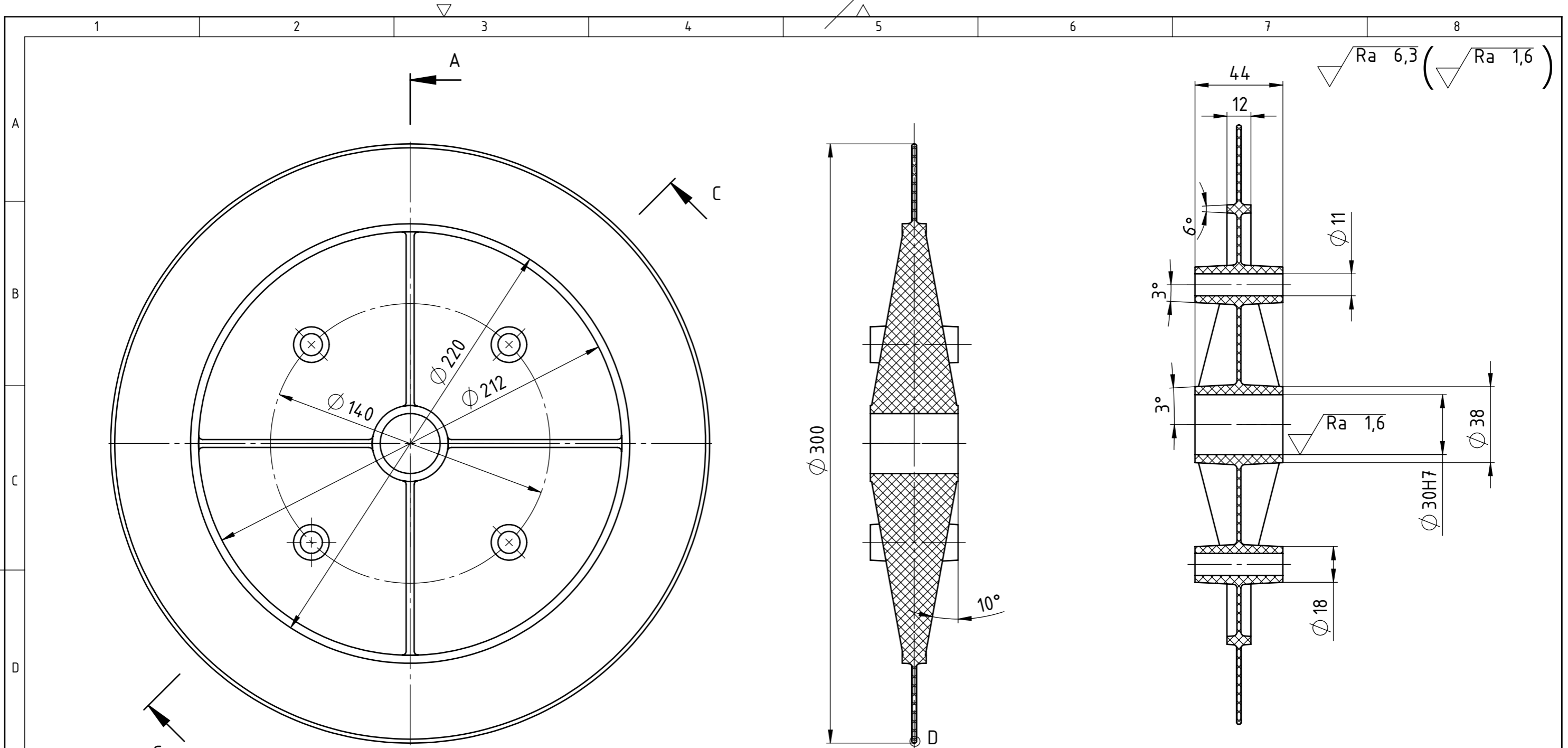
C-C M(1:2)
