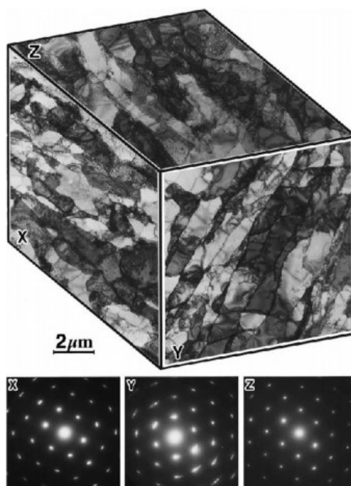
Slika 31. Mikrostruktura polikristalnog aluminija nakon jednog prolaza ECAP-a i SAED uzorci [10]
