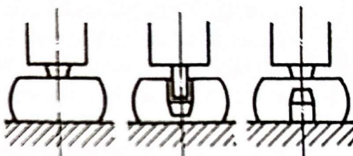
Slika 23. Probijanje [6]
