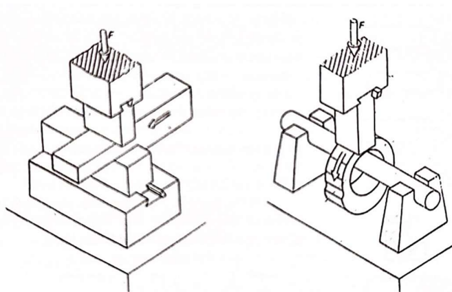
Slika 22. Postupak iskivanja [6]
