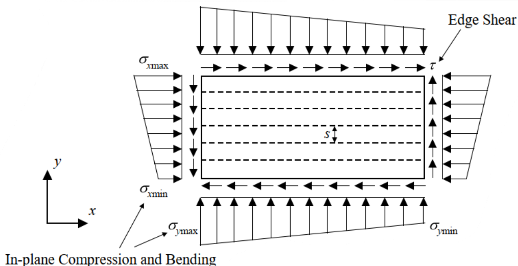
Slika 6-22 Moguća raspodjela naprezanja na ukrepljenom panelu [22]
