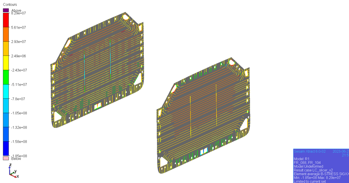
Slika- C-XIV Aksijalna napreznaja u grednim konačnim elementima na vodonepropusnim poprečnim pregradama (rebro br. 88 i 104) [MPa]
