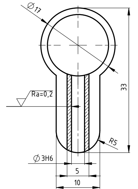
Presjek: F-F
