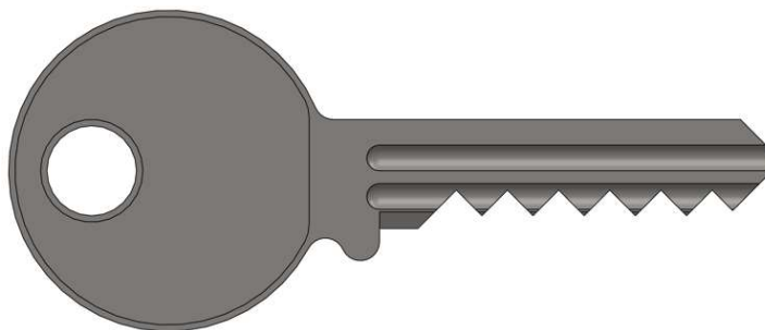
Slika 12.7 - Ključ brušen na najdublje zarezke, za napad udaranjem
