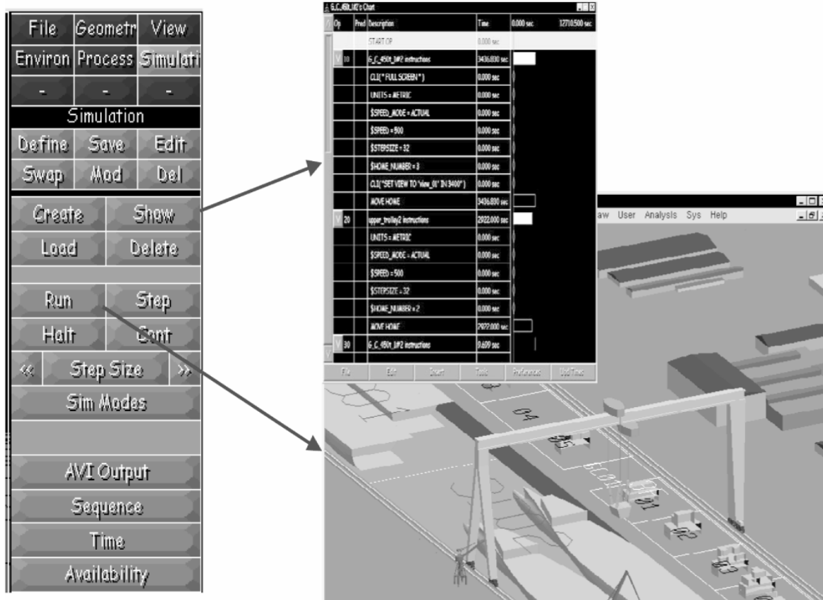
Slika 55 Pokretanje simulacije [27]
