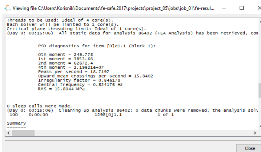
Slika 36. Parametri za dobivanje rezultata u frekvencijskoj domeni
