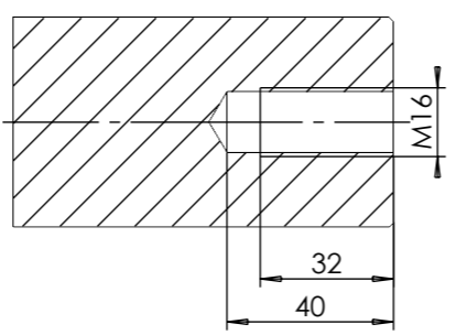
Presjek D-D M1:2
