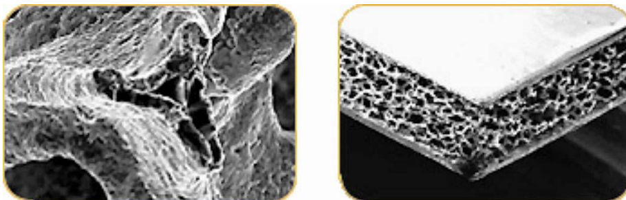
Slika 4.13. Sendvič-konstrukcija s jezgrom od niklene pjene [1]
