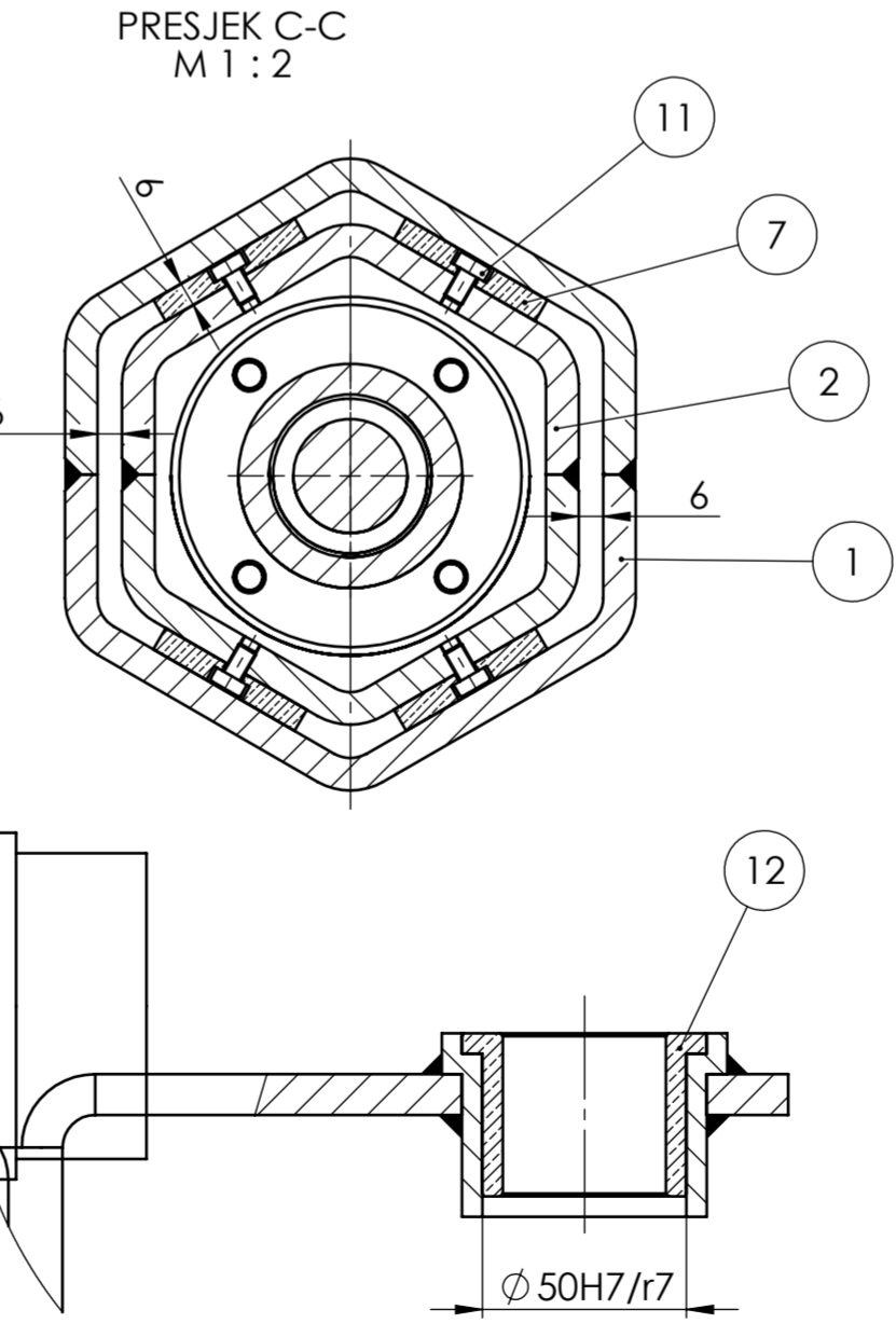
DETALJ Z M 1:2
