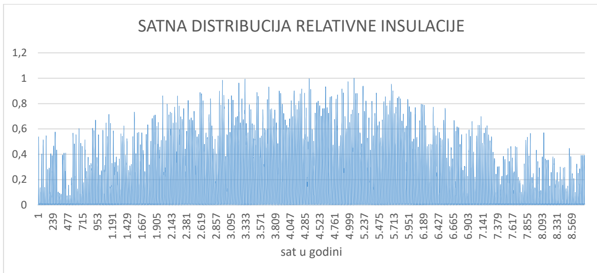
Slika 32. Kvalitativna krivulja satne insulacije.
