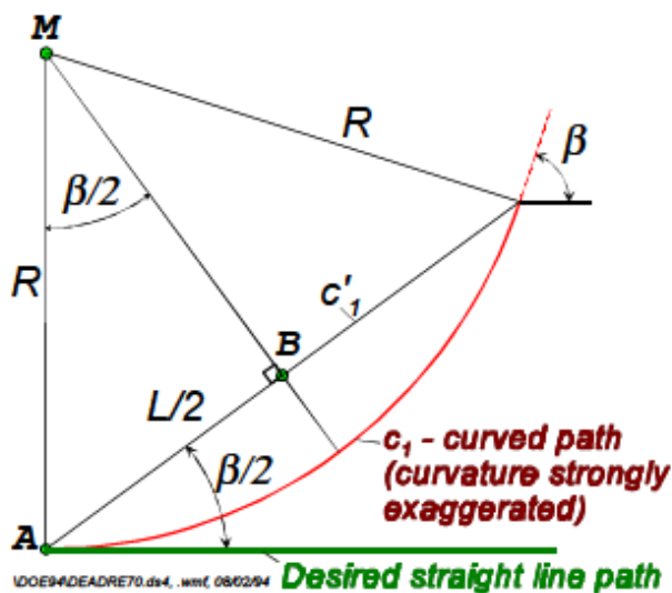
Slika 41. ABM trokut za izračun polumjera zakrivljenosti kretnje robota [12]
