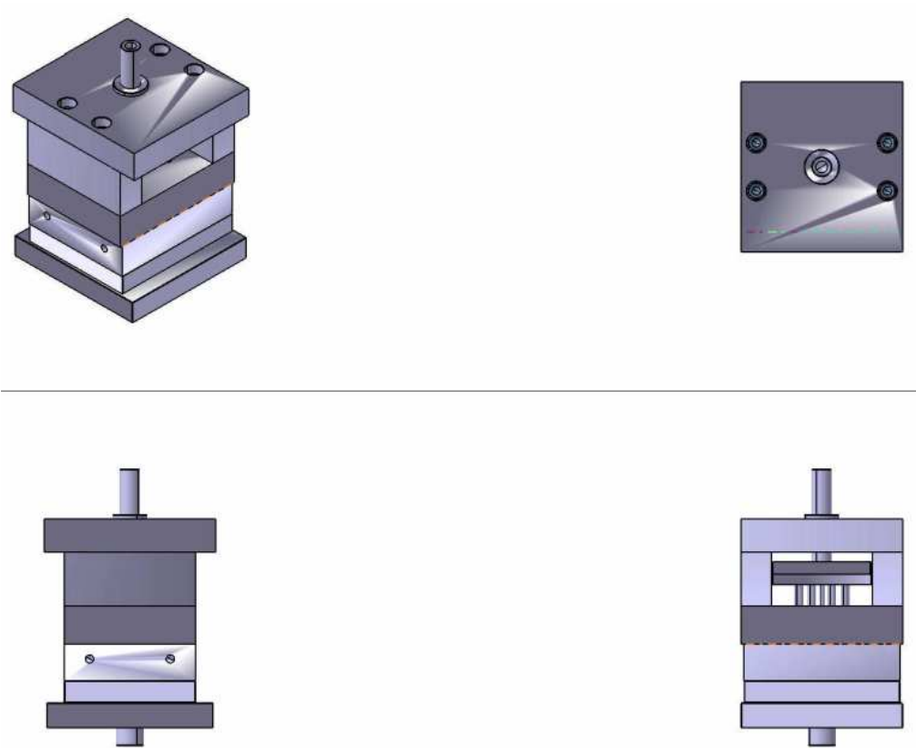
Slika 4.10. Kalup
