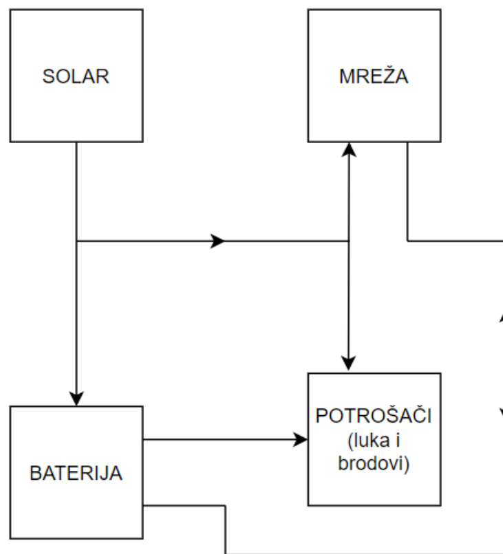
Slika 6 Shema toka električne energije
