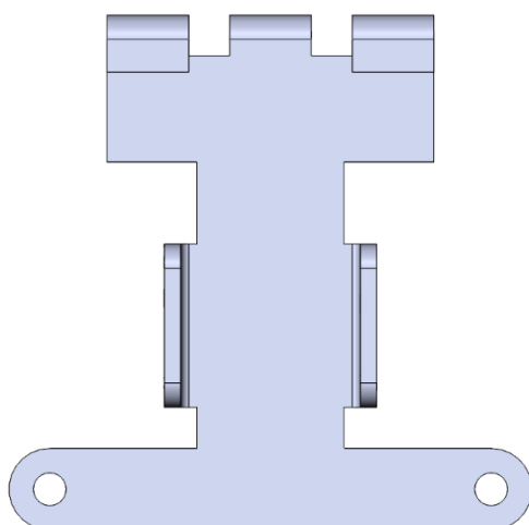
Slika 76. Prikaz glavnog lima u nacrtu (lijevo) i izometriji (desno)
