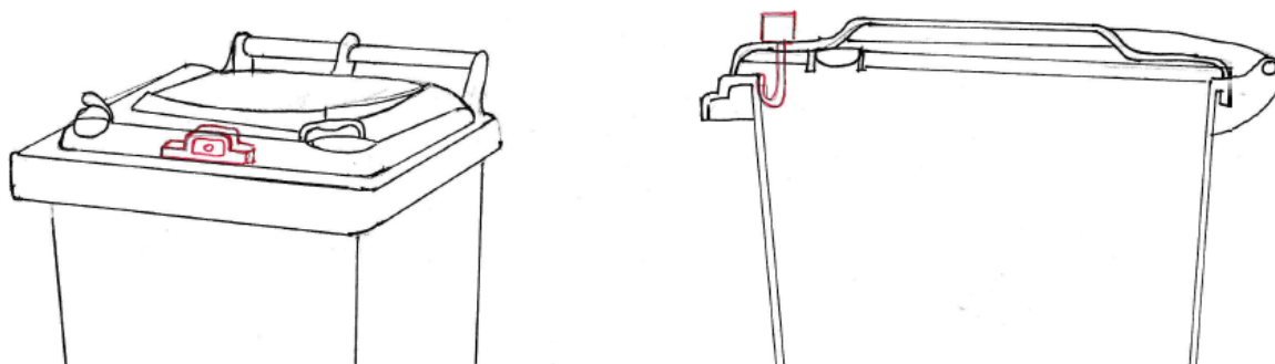
Slika 26. Prikaz prihvaćanja koncepta 4 na spremnik izvana (lijevo) i u presjeku (desno)
