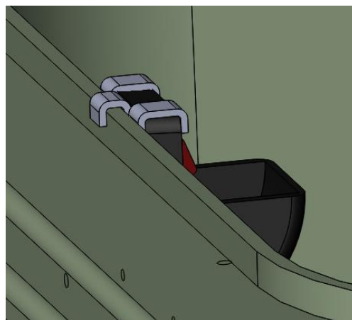
Slika 74. Prikaz hvatanja donjeg sklopa na spremnik pomoću zakrivljenog dijela lima
