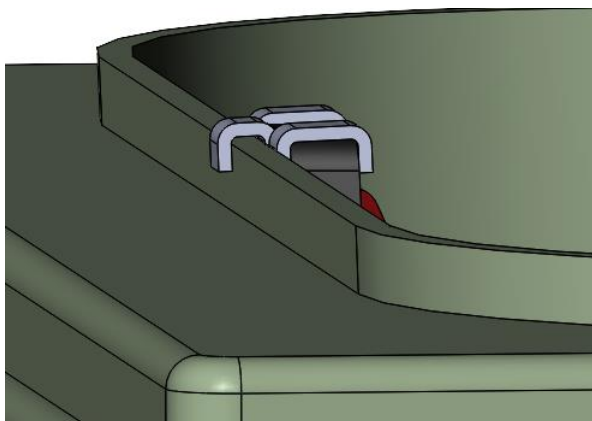
Slika 74. Prikaz hvatanja donjeg sklopa na spremnik pomoću zakrivljenog dijela lima
