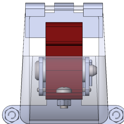
Slika 75. Prikaz unutrašnjih komponenti donjeg dijela sklopa u izometriji (lijevo) i nacrtu (desno)
