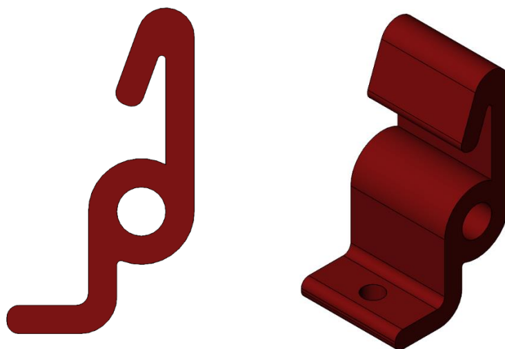
Slika 77. Prikaz "kuke" u bocrtu (lijevo) i izometriji (desno)
