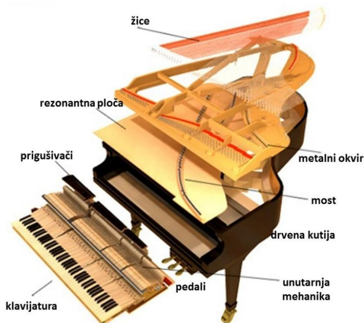
Slika 3. Eksplozirani prikaz građe suvremenog klavira [3]
