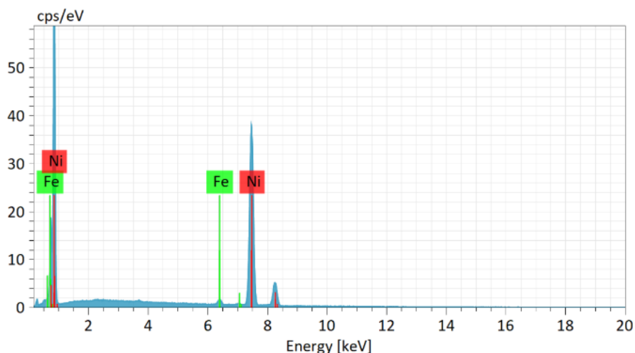
Slika 38: EDX spektar dobiven analizom prevlake
