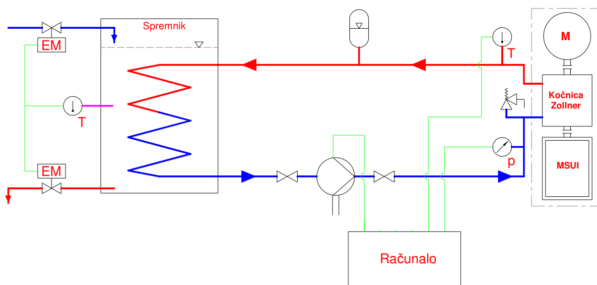
Slika 5.11. Shema rada i toka informacija koncepta II
