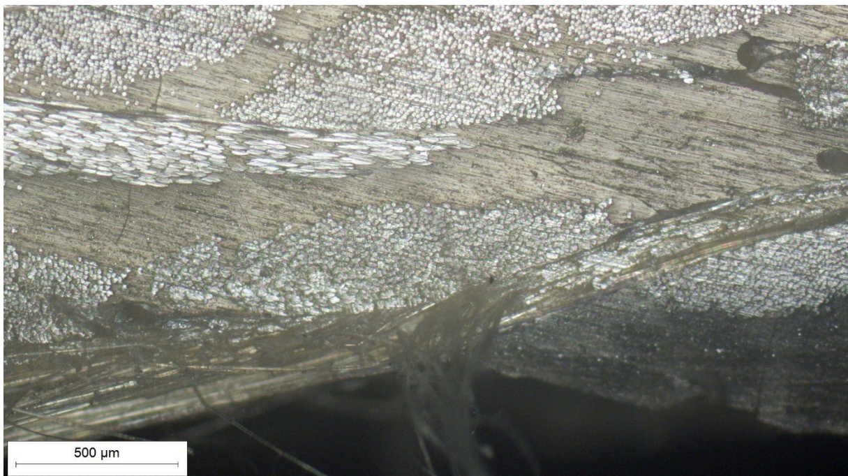
Slika 30. Presjek A uzorka na mjestu udara zrna (50:1, pozadina)
