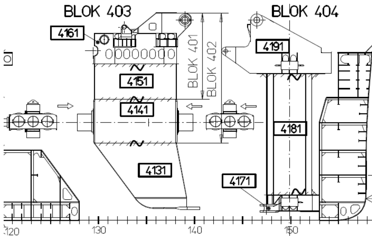
Slika 32. : Prikaz karakterističnih sekcija okretnog pramca
