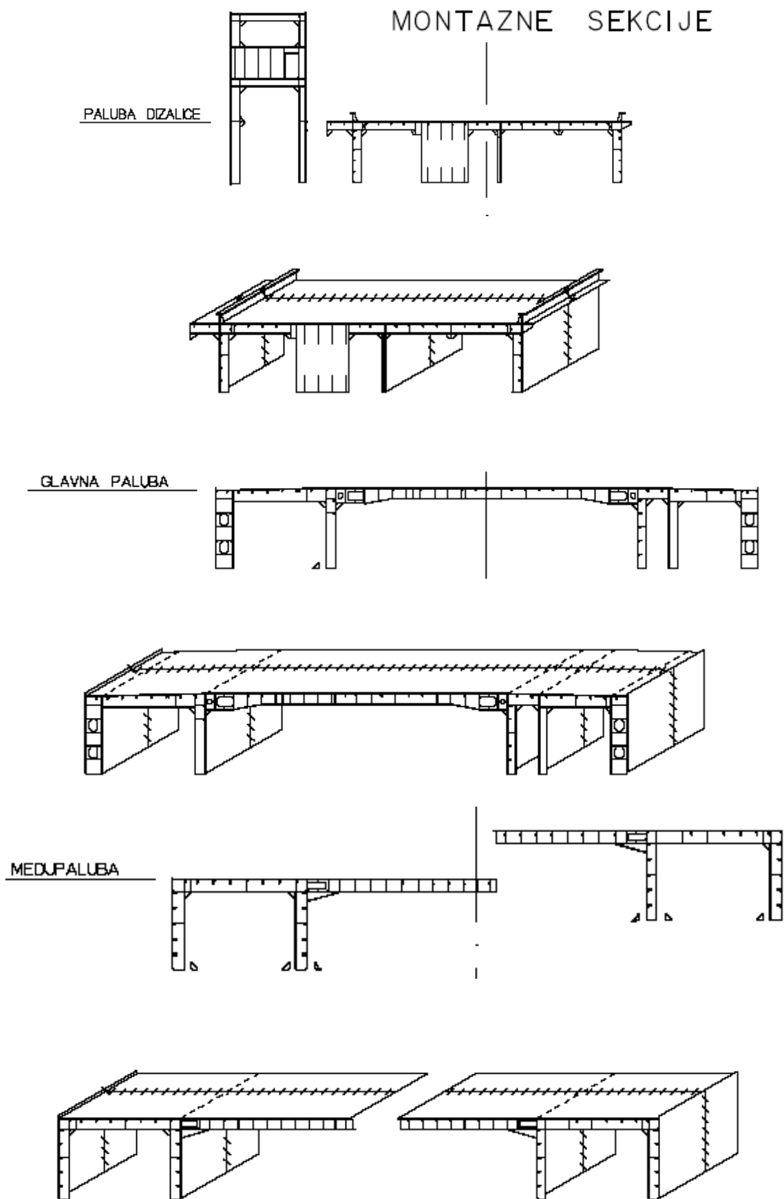
Slika 29. : Prikaz montažnih sekcija palube dizalice, glavne palube, međupalube i krova dvodna
