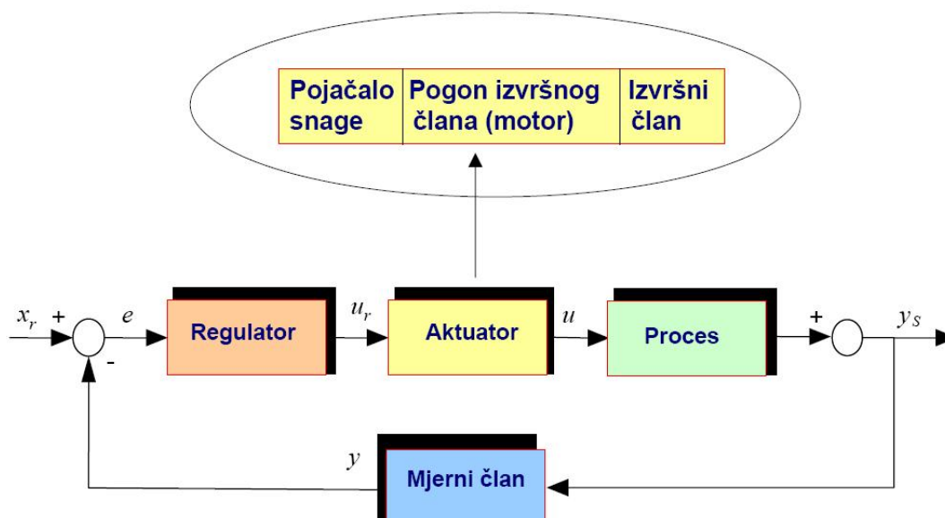
Slika 3.1. Komponente aktuatora [13]
