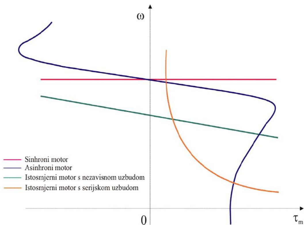
Slika 3.2. Mehaničke karakteristike motora [13]
