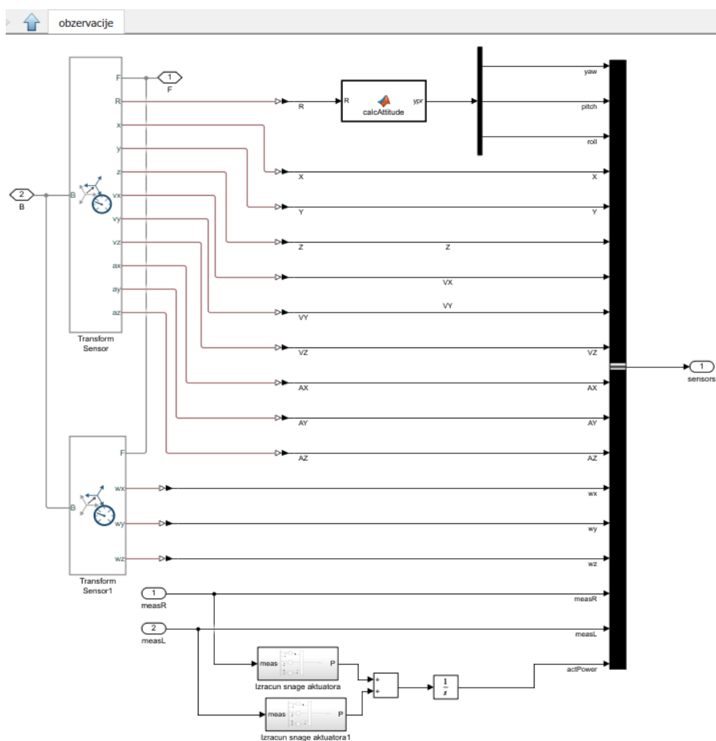
Slika 44 Blok “obzervacije“
