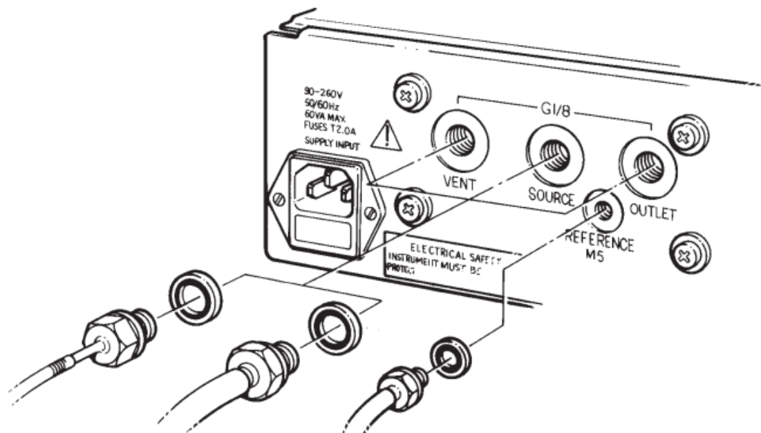
Slika 31. Pneumatski priključci
