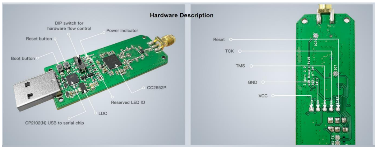
Slika 28. Zigbee dongle
