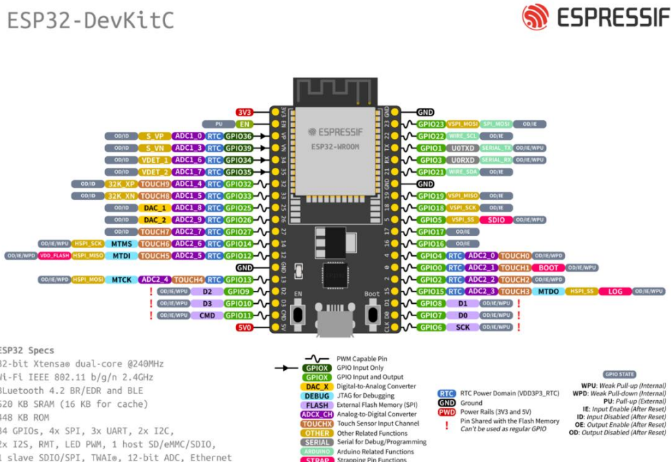
Slika 35. Izgled i "pinout" ESP32
