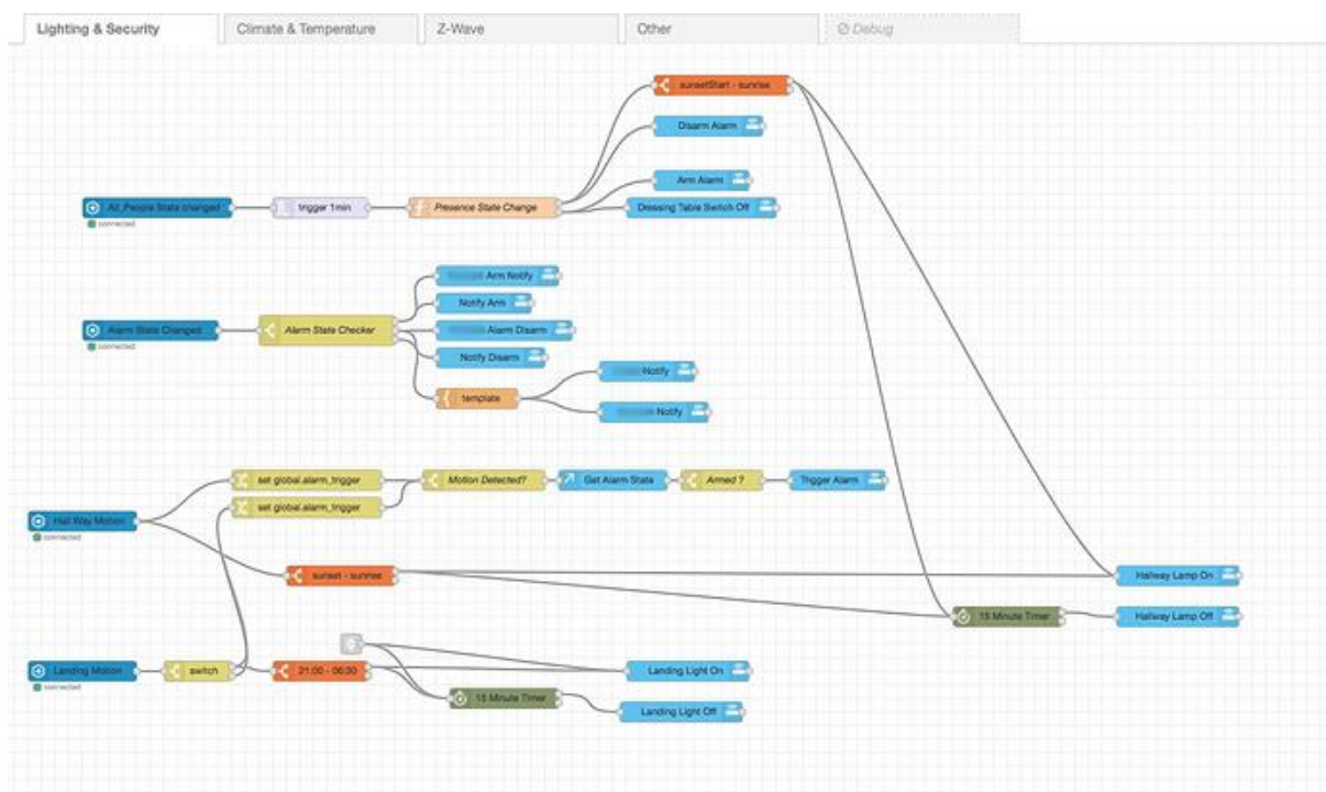
Slika 59. Node-RED programiranje
