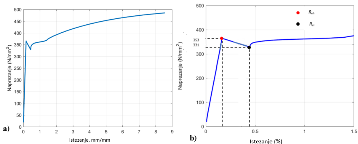
Slika 40. \sigma - \epsilon dijagram (a) s istaknutim područjem elastičnosti (b) za frekvenciju ispitivanja 1 Hz, čelik C15E
