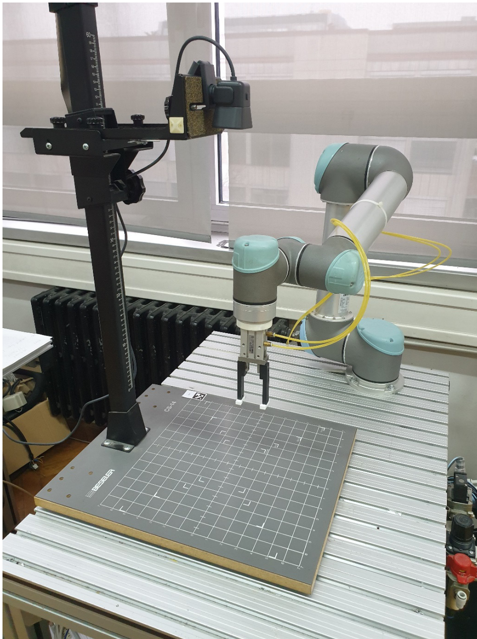
Slika 7.1. Radni postav
