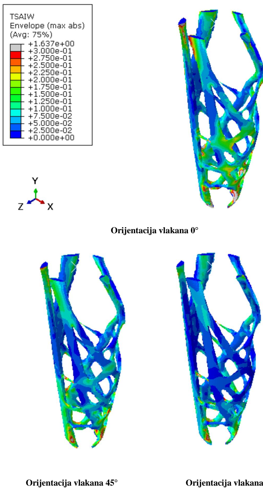
Slika 51. Rezultati topološki optimirane proteze potkoljenice: Tsai – Wu kriterij popuštanja [-]
