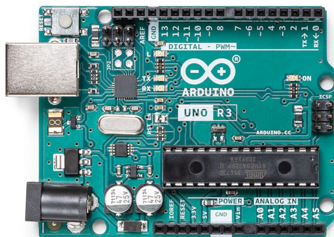
Slika 49. Mikrokontroler Arduino Uno Rev3 [28]
