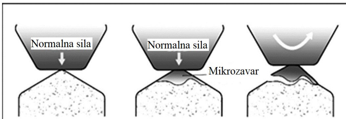
Slika 11. Nastanak adhezijskog trošenja [8]
